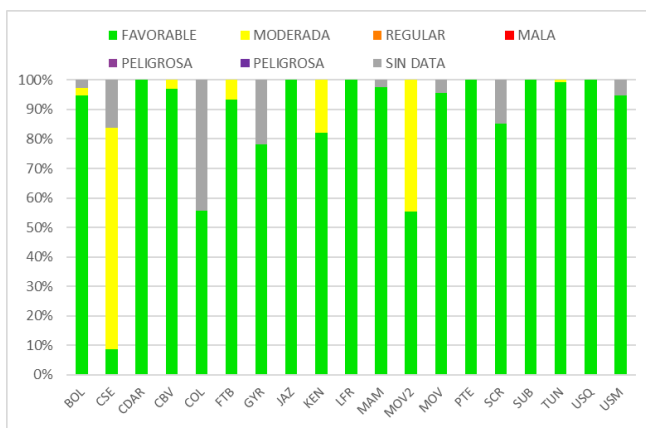
Figura 20. IBOCA para PM 10 por estación - septiembre 2021
