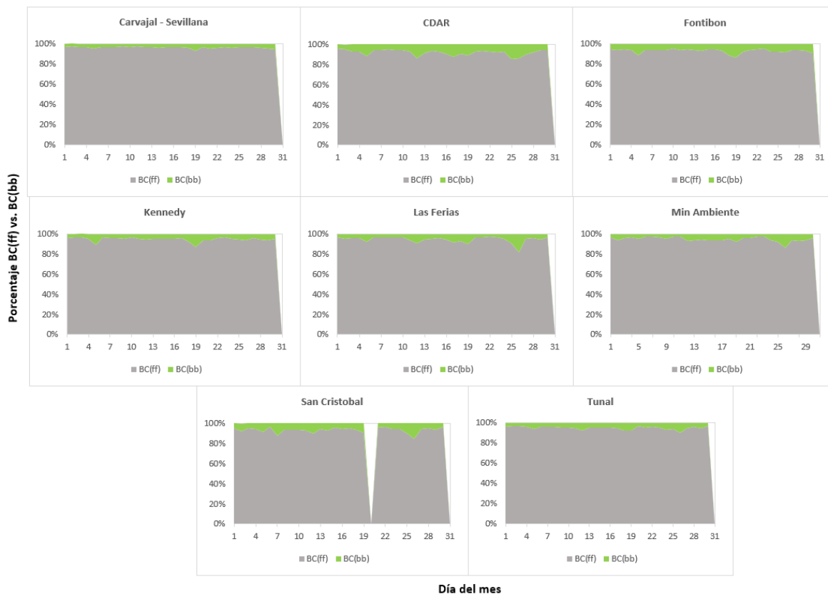
Figura 19. Serie temporal porcentaje de quema Black Carbon de combustibles fósiles BC(ff) vs. Black Carbon de quema de biomasa BC(bb) - septiembre 2021
