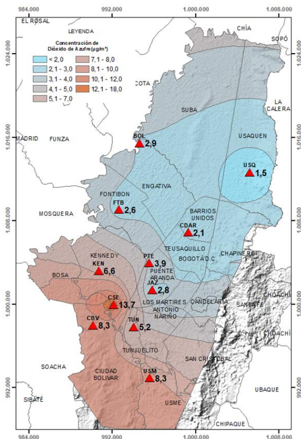
Figura 12. Distribución espacial concentraciones mensuales SO 2 - septiembre 2021
