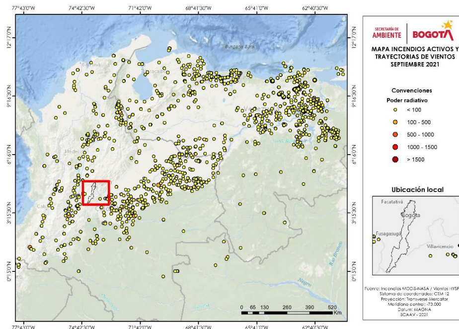
Figura 17. Distribución espacial de incendios activos identificados por el sensor MODIS en el mes de septiembre 2021
