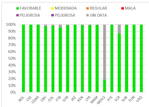
Figura 22. IBOCA para O 3 por estación - septiembre 2021
