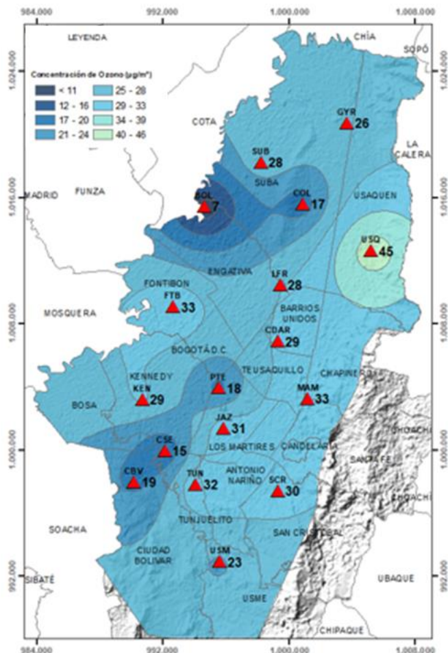
Figura 10. Distribución espacial concentraciones mensuales O 3 - septiembre 2021
