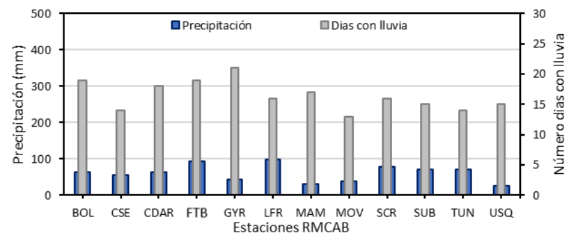
Figura 26. Precipitación media mensual y número de días con precipitación – septiembre 2021
