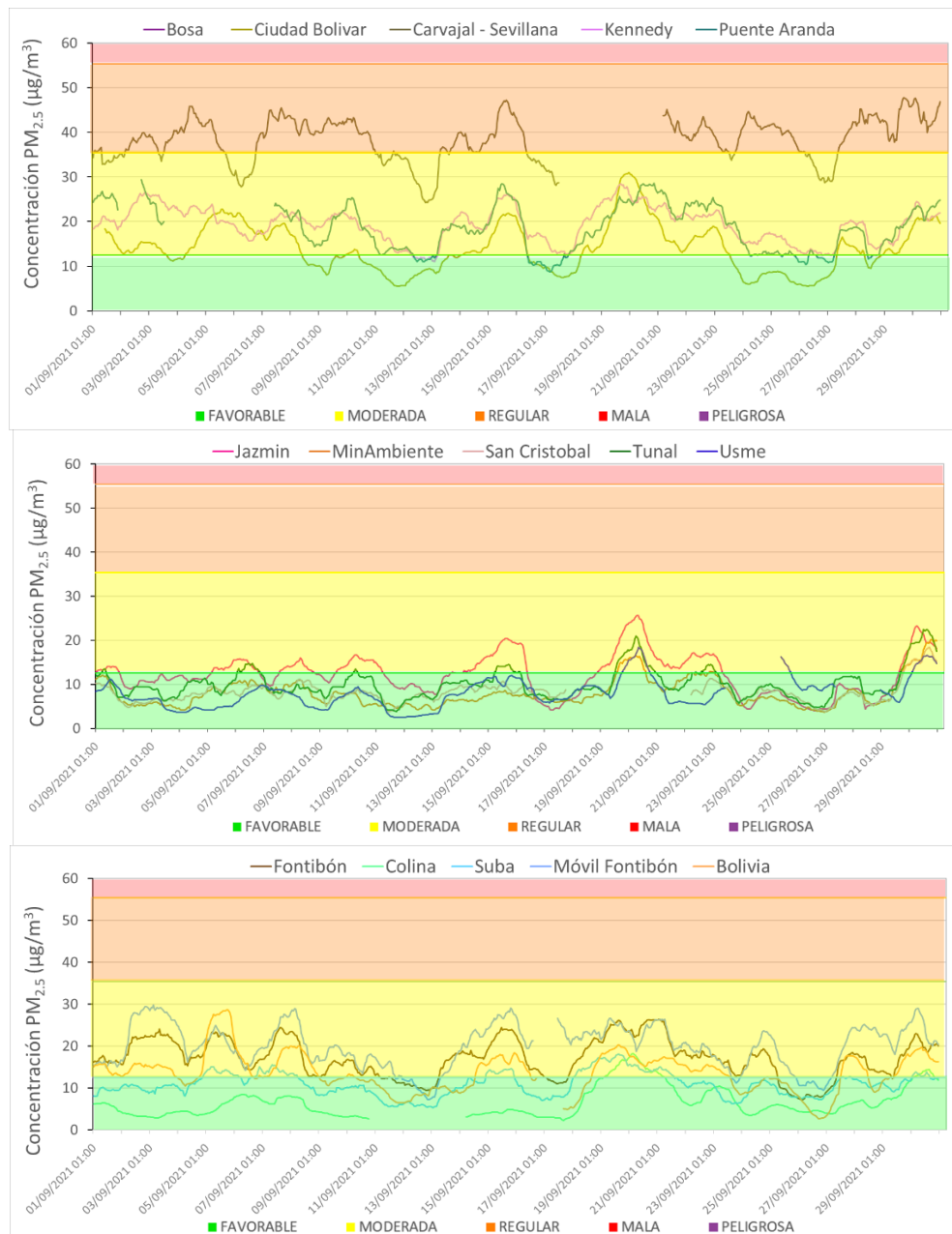
Figura 23. Concentraciones media móvil 24 h PM_{2.5} septiembre 2021
