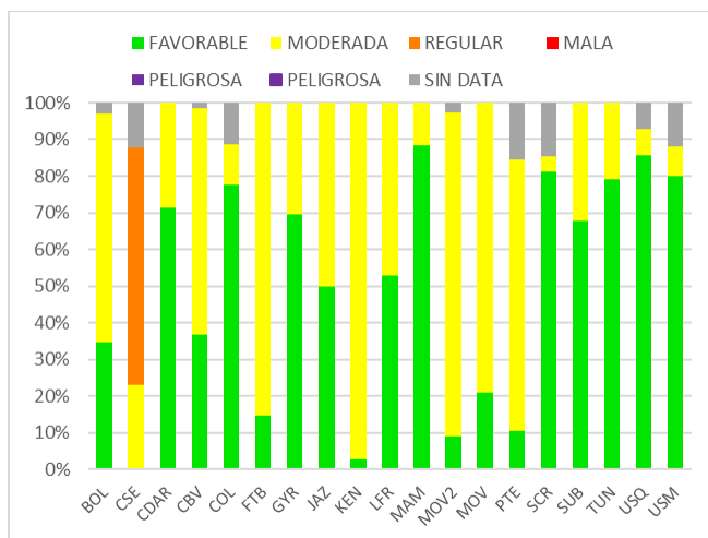
Figura 21. IBOCA para PM 2.5 por estación - septiembre 2021
