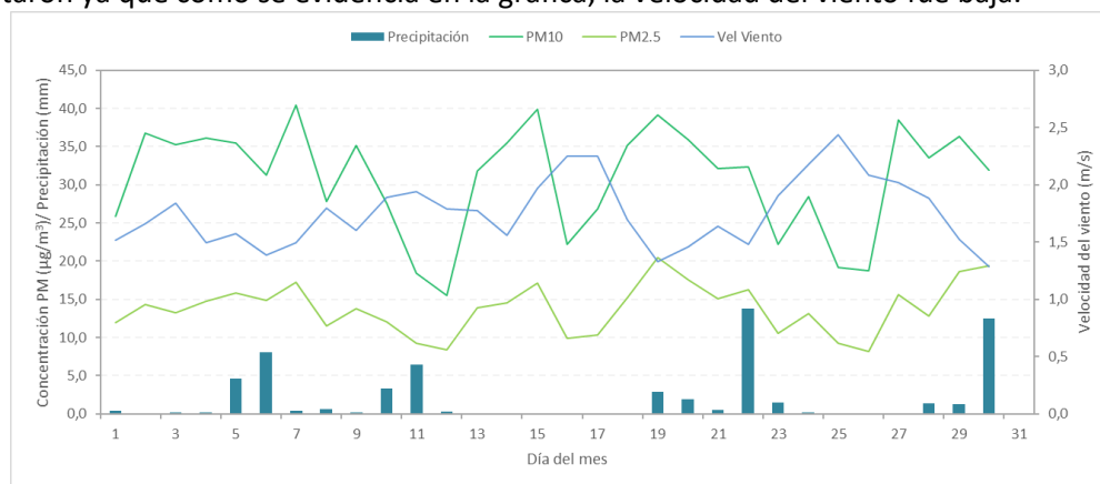
Figura 6. Promedio de concentración PM_{10} y PM_{2.5} , precipitación y velocidad del viento a nivel ciudad - septiembre 2021
