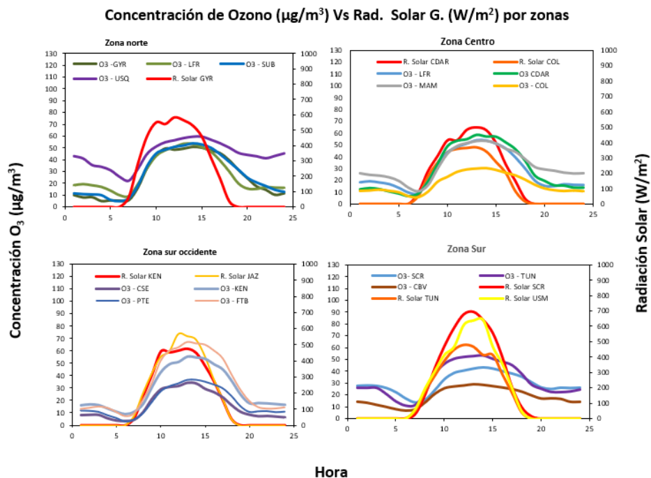
Figura 11. Comportamiento horario de las concentraciones de \text{O}_3 ( \mu\text{g}/\text{m}^3 ) y su relación con la Radiación Solar entrante ( \text{W}/\text{m}^2 ) - Septiembre 2021. a) zona norte, b) zona centro, c) zona suroccidente y d) zona sur
