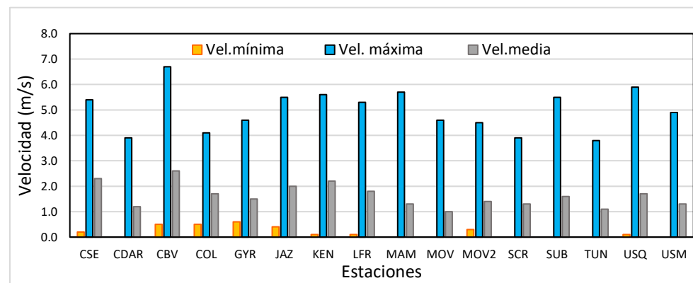
Figura 30. Velocidad del viento media, máxima y mínima absolutas por estación - septiembre 2021.
