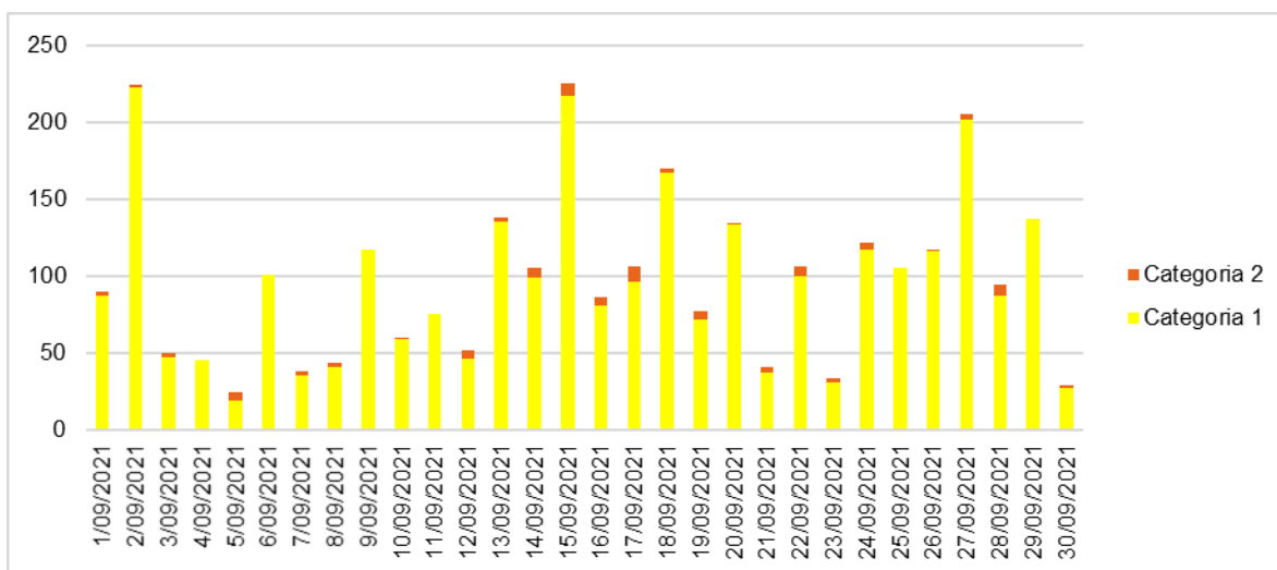
Figura 18. Número de eventos o puntos calientes identificados por el sensor MODIS en el mes de septiembre 2021
