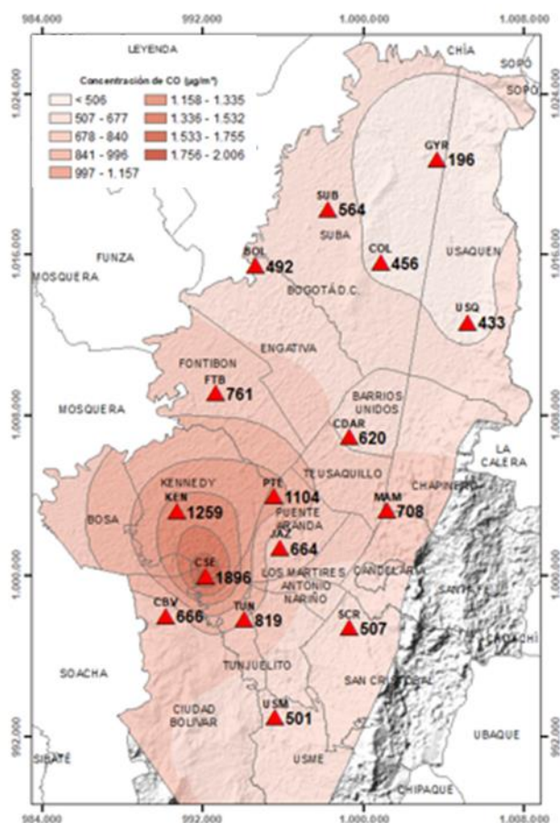
Figura 14. Distribución espacial concentraciones mensuales CO - septiembre 2021.
