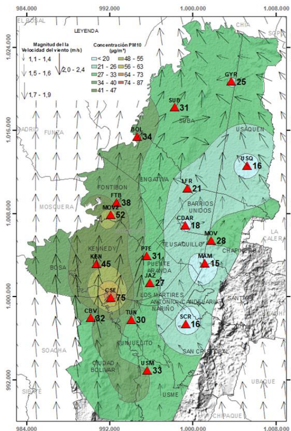
Figura 2. Distribución espacial concentraciones mensuales PM 10 - septiembre 2021
