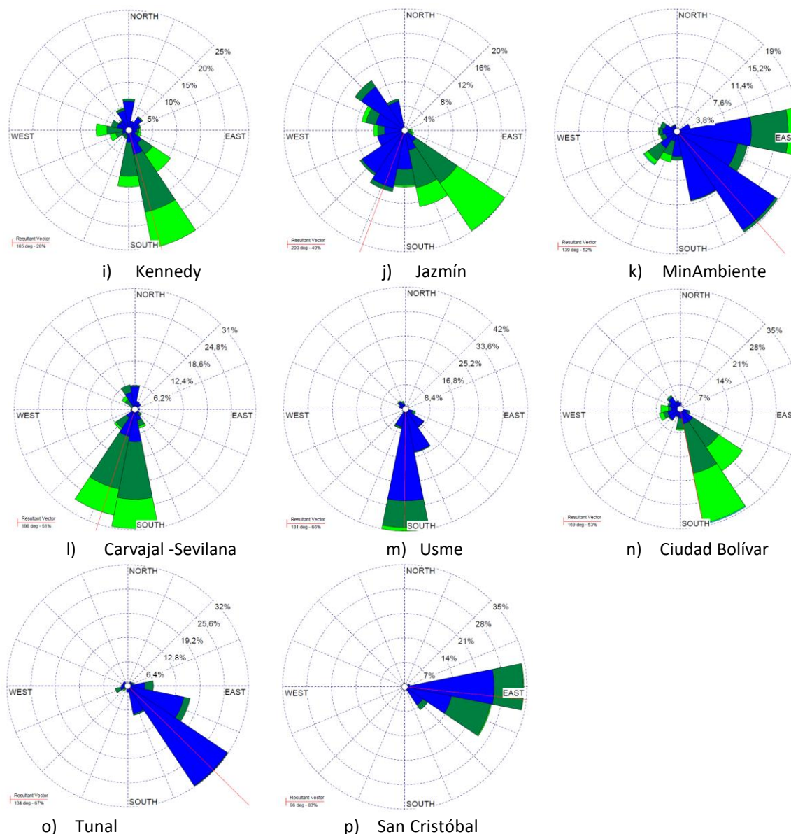
Figura 31. Rosas de los vientos – septiembre 2021
