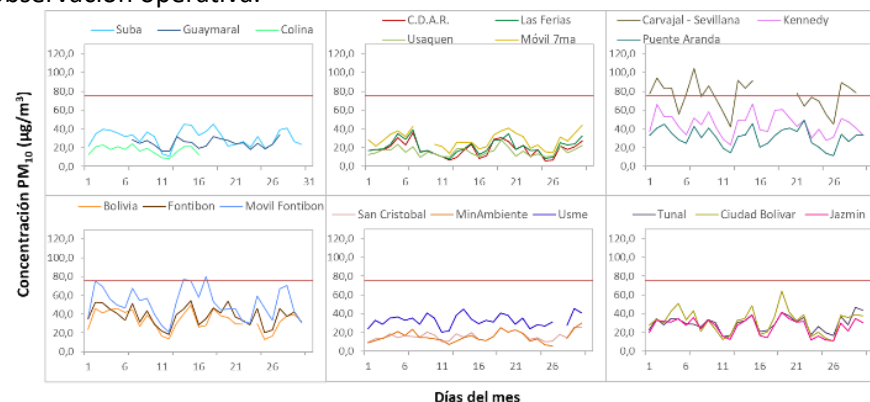
Figura 3. Concentraciones diarias PM 10 por estación de monitoreo - septiembre 2021
