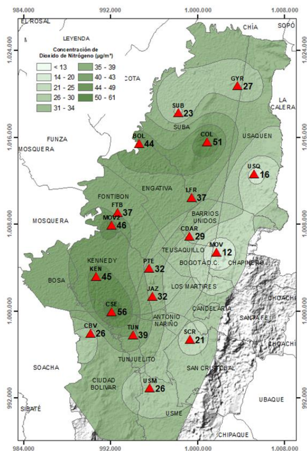
Figura 13. Distribución espacial concentraciones mensuales NO 2 - septiembre 2021
