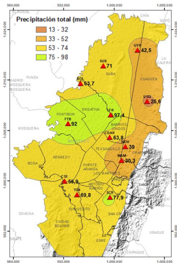
Figura 25. Mapa de la precipitación mensual total (mm) - septiembre 2021.
