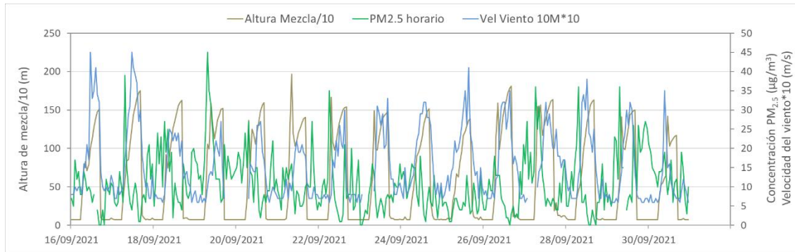
Figura 8. Comparación altura de mezcla, concentraciones PM_{2.5} y velocidad del viento estación Guaymaral septiembre 2021
