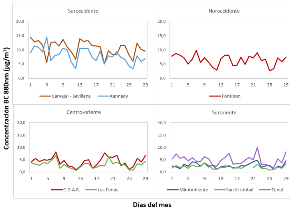
Figura 16. Comportamiento de las concentraciones diarias de longitud de onda 880nm para septiembre de 2021
