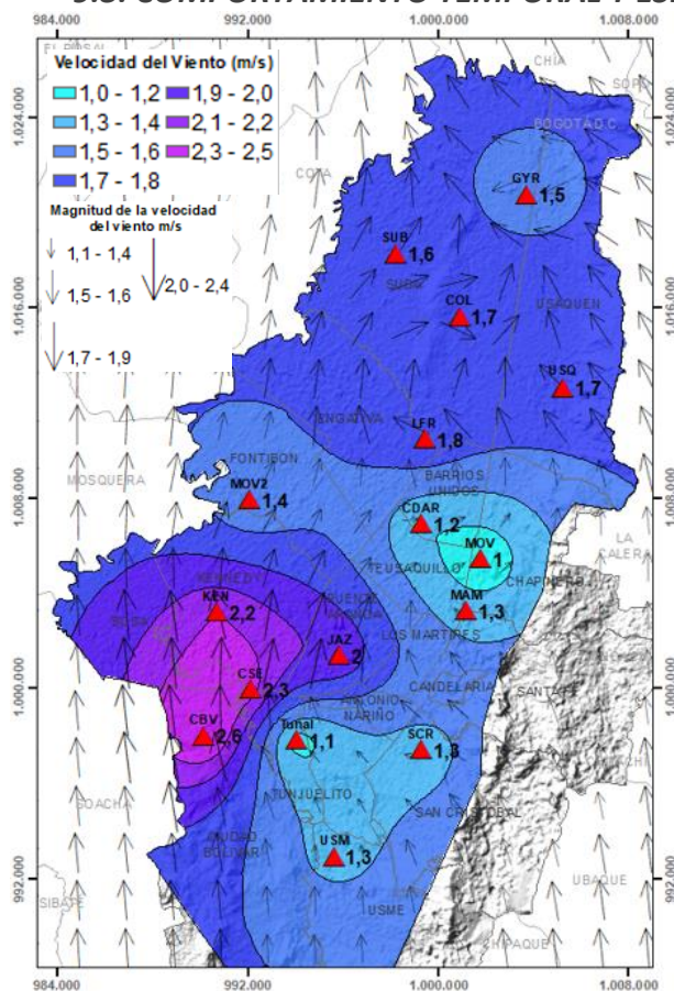
Figura 29. Velocidad promedio (Superficie en colores) y Dirección promedio (Vectores) del Viento de Bogotá con base en la interpolación de Kriging -septiembre 2021
