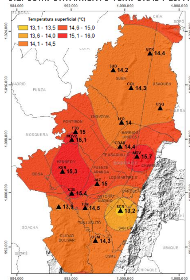
Figura 27. Mapa del promedio de temperatura superficial de las estaciones de la RMCAB con base en el método de interpolación de Kriging – septiembre 2021
