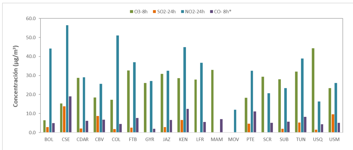
Figura 9. Concentraciones mensuales de gases (O 3 , SO 2 , NO 2 y CO) por estación de monitoreo - septiembre 2021
