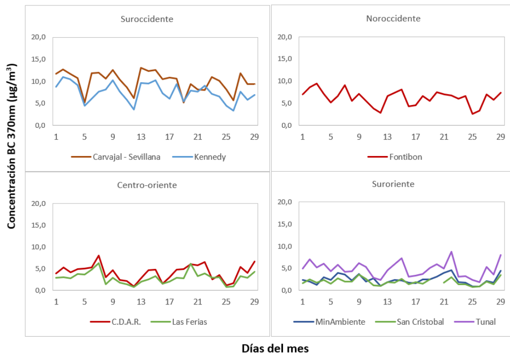
Figura 15. Comportamiento de las concentraciones diarias de longitud de onda 370nm para septiembre de 2021
