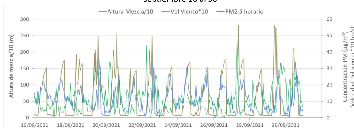
Figura 7. Comparación altura de mezcla, concentraciones PM 2.5 y velocidad del viento estación Tunal - septiembre 2021
