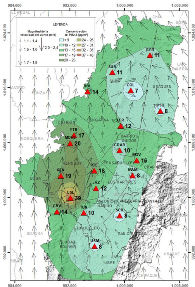
Figura 4. Distribución espacial concentraciones mensuales PM 2.5 - septiembre 2021.
