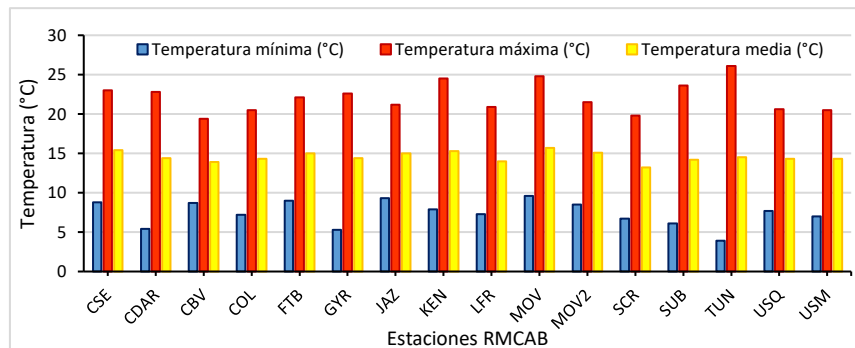
Figura 28. Temperaturas medias, máximas y mínimas absolutas por estación - septiembre 2021
