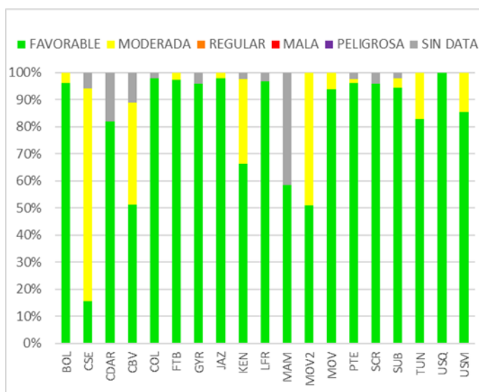
Figura 22. IBOCA para PM 10 por estación – octubre 2023
