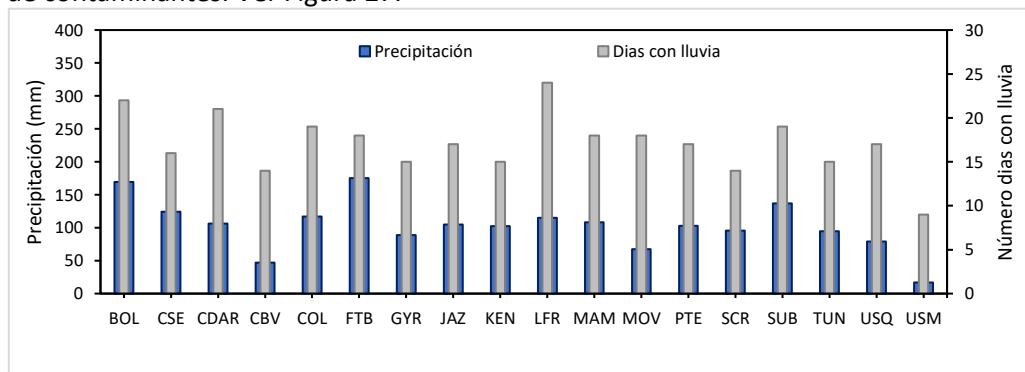
Figura 27. Precipitación media mensual y número de días con precipitación – octubre 2023
