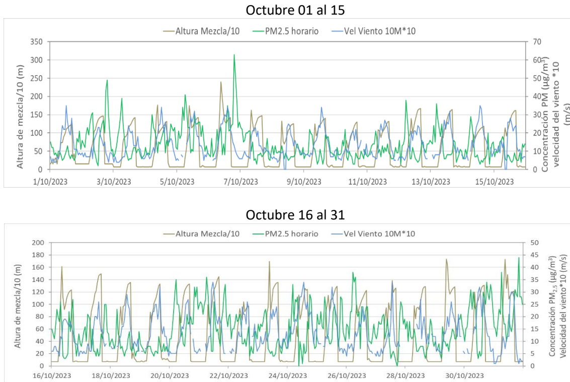
Figura 8. Comparación altura de mezcla, concentraciones PM_{2.5} y velocidad del viento estación Guaymaral - octubre 2023
