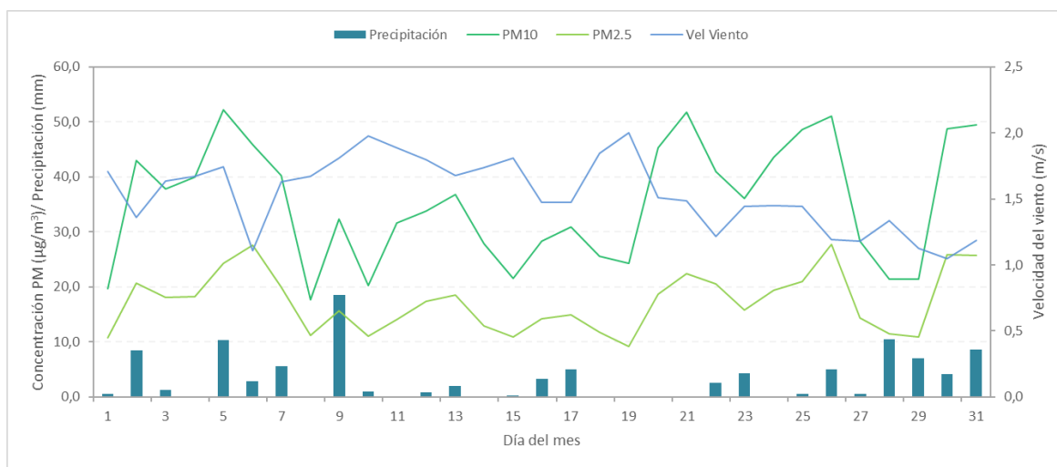
Figura 6. Promedio de concentración PM 10 y PM 2.5 , precipitación y velocidad del viento a nivel ciudad – octubre 2023
