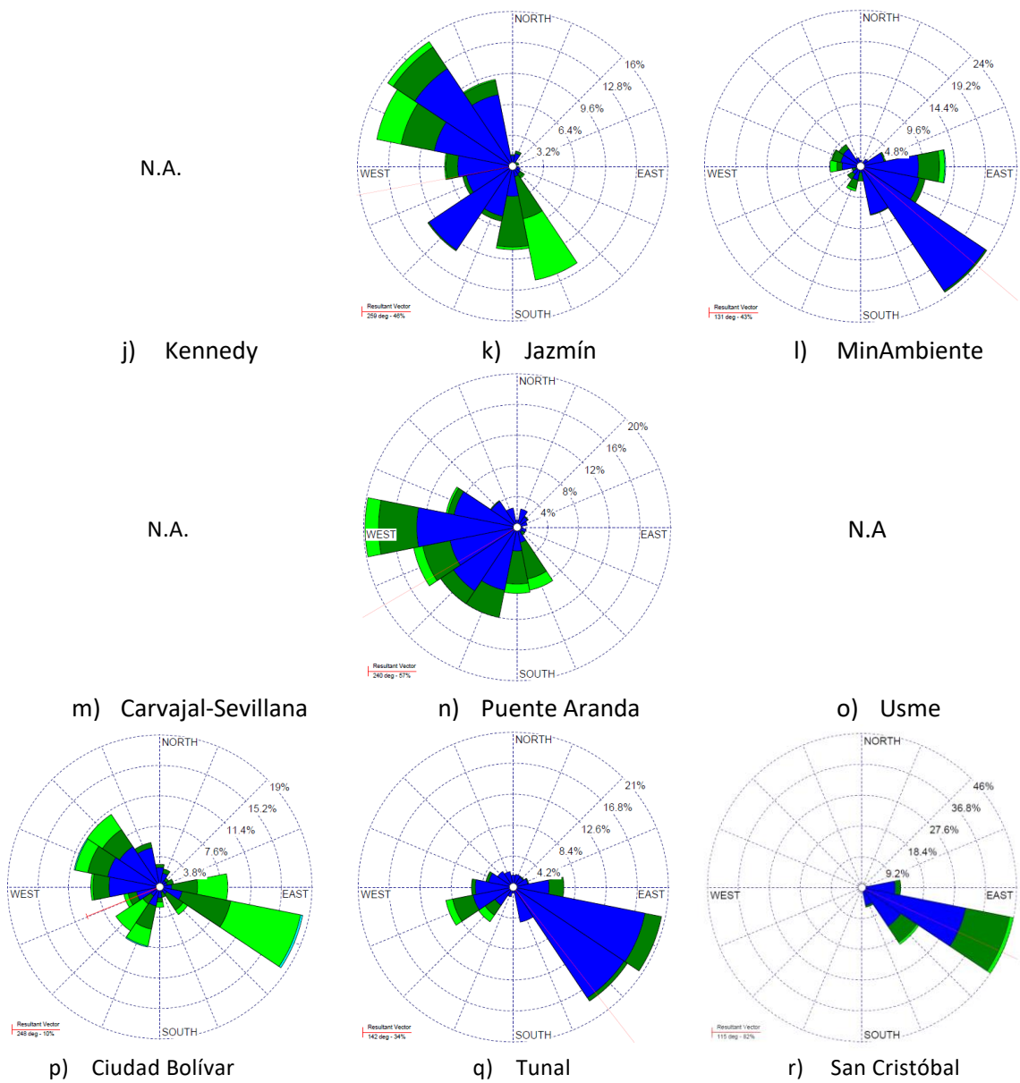
Figura 32. Rosas de los vientos – octubre de 2023
