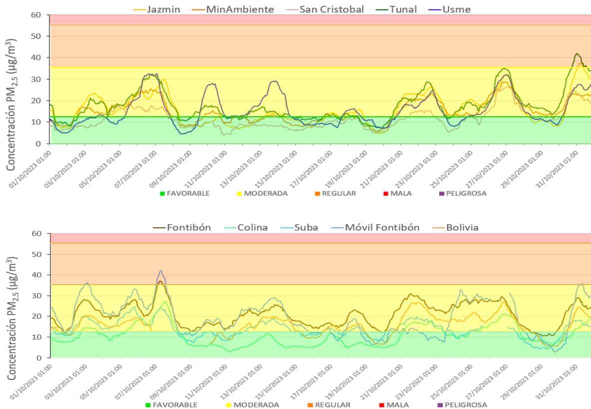
Figura 25. Concentraciones media móvil 24 h PM 2.5 octubre 2023
