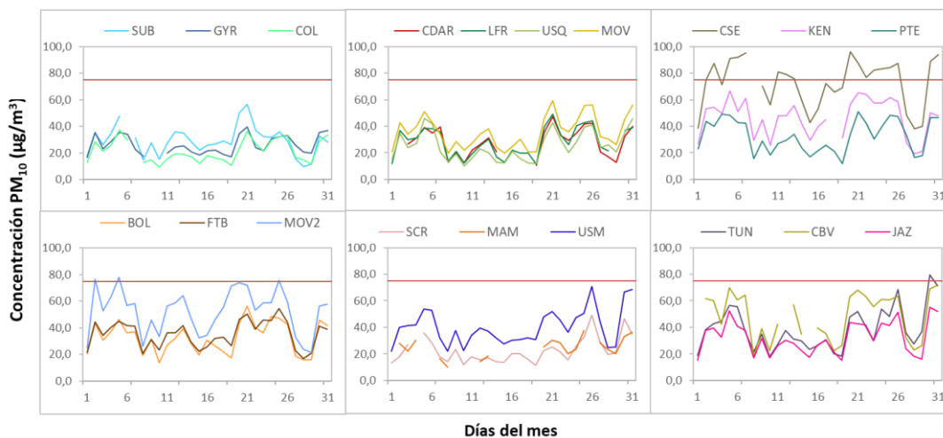
Figura 3. Concentraciones diarias PM 10 por estación de monitoreo - octubre 2023
