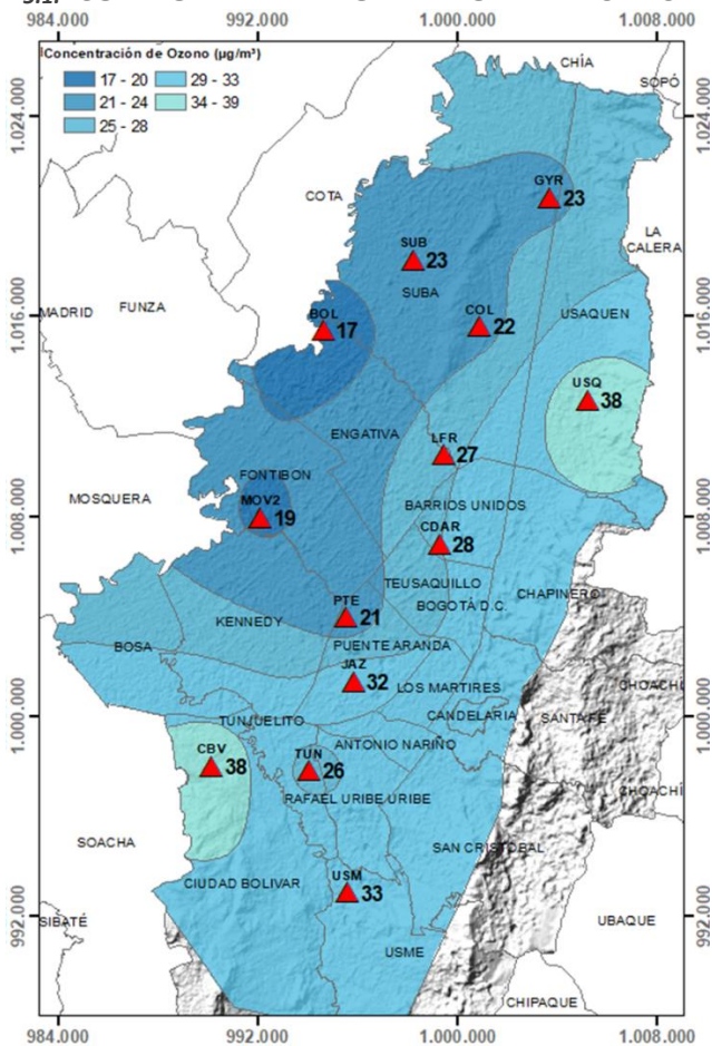
Figura 10. Distribución espacial concentraciones mensuales O 3 – octubre 2023
