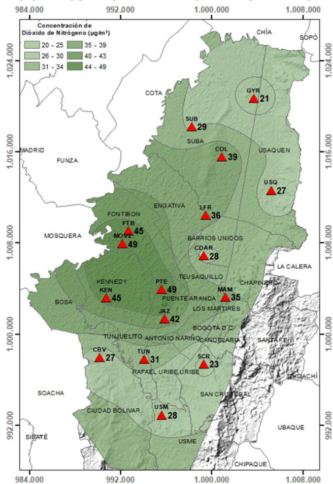
Figura 15. Distribución espacial concentraciones mensuales NO 2 - octubre 2023
