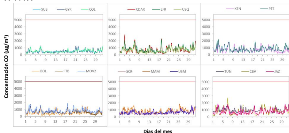
Figura 18. Concentraciones media móvil 8 horas de CO por estación de monitoreo - octubre 2023
