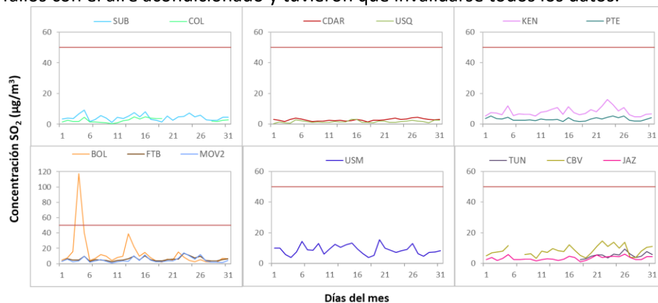
Figura 14. Concentraciones promedio mensuales de SO 2 por estación de monitoreo - octubre 2023
