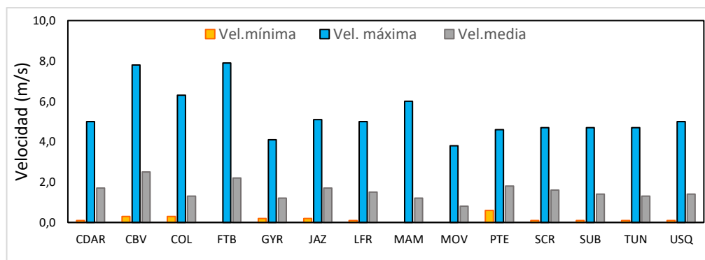
Figura 31. Velocidad del viento media, máxima y mínima absolutas por estación – octubre 2023
