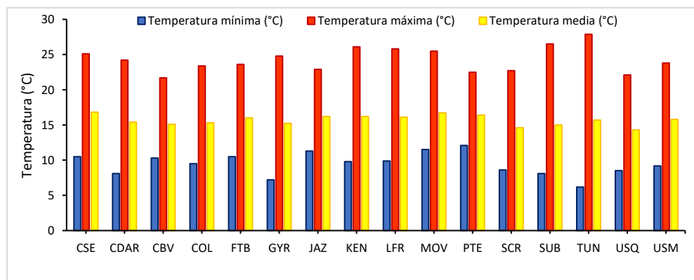
Figura 29. Temperaturas medias, máximas y mínimas absolutas por estación – octubre 2023
