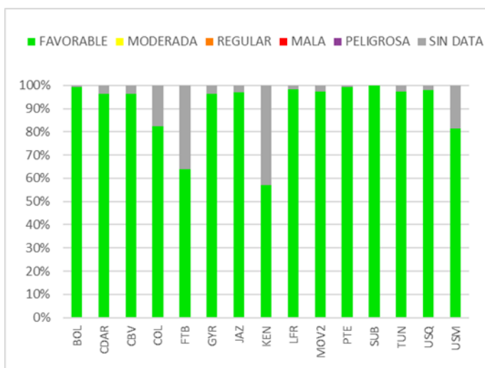
Figura 24. IBOCA para O 3 por estación – octubre 2023
