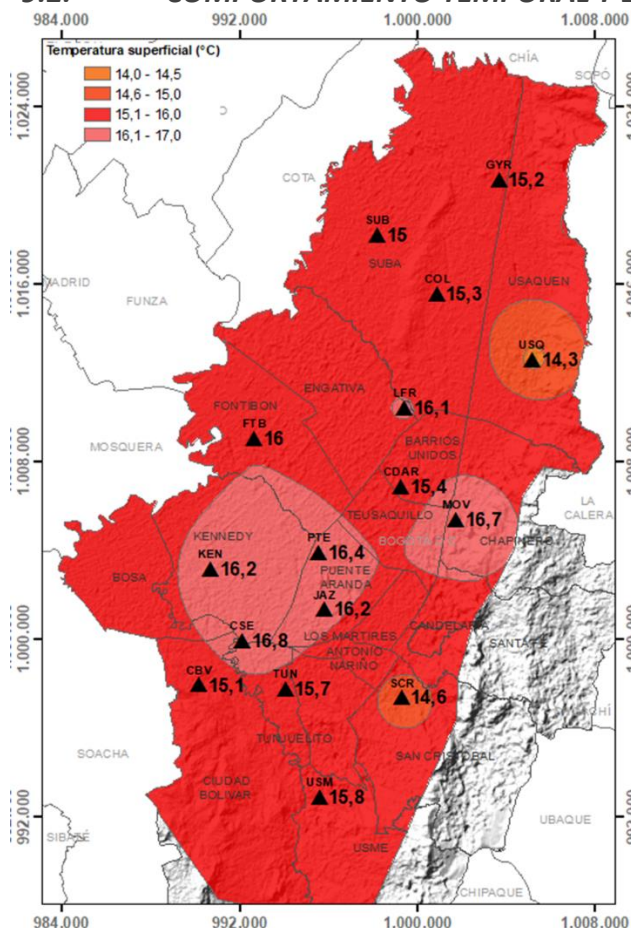
Figura 28. Mapa del promedio de temperatura superficial de las estaciones de la RMCAB con base en el método de interpolación de Kriging – octubre 2023
