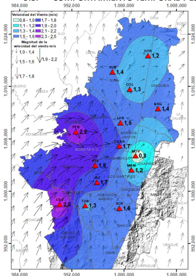
Figura 30. Velocidad promedio (Superficie en colores) y Dirección promedio (Vectores) del Viento con base en Kriging – octubre 2023
