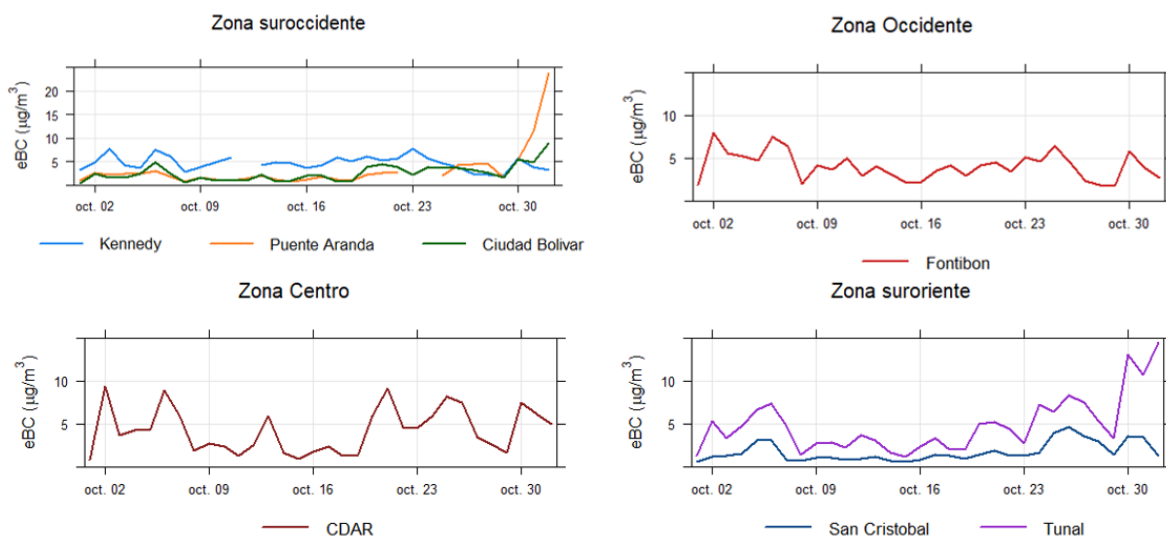
Figura 19. Comportamiento de las concentraciones diarias de eBC para octubre de 2023
