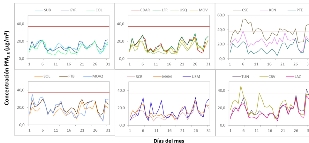
Figura 5. Concentraciones diarias PM 2.5 por estación de monitoreo – octubre 2023
