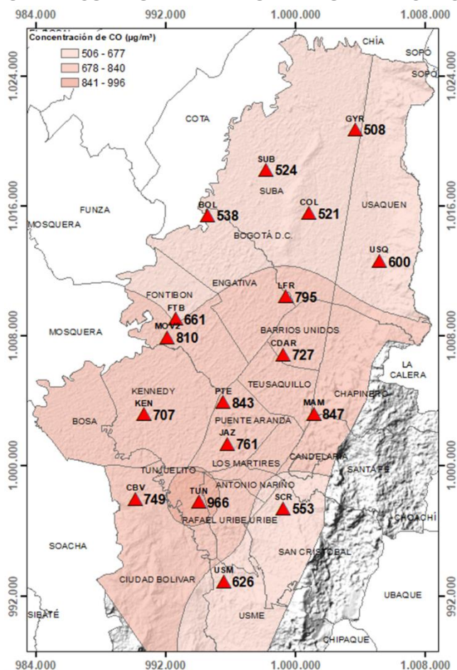
Figura 17. Distribución espacial concentraciones mensuales CO – octubre 2023
