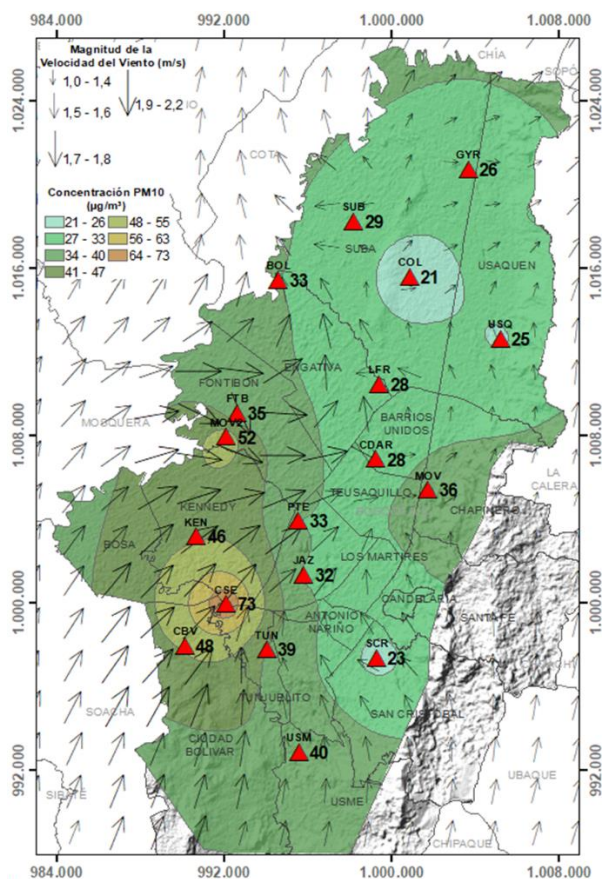
Figura 2. Distribución espacial concentraciones mensuales PM 10 – octubre 2023
