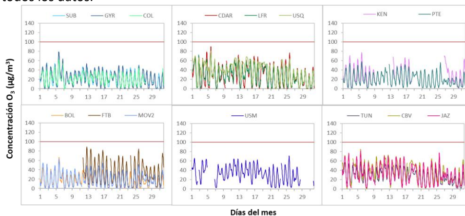
Figura 11. Concentraciones media móvil 8 horas de O 3 por estación de monitoreo - octubre 2023
