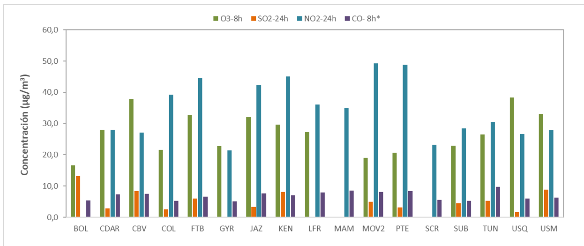
Figura 9. Concentraciones mensuales de gases (O 3 , SO 2 , NO 2 y CO) por estación de monitoreo - octubre 2023
