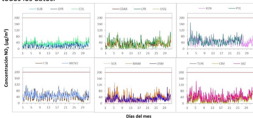
Figura 16. Concentraciones promedio mensuales de NO 2 por estación de monitoreo - octubre 2023
