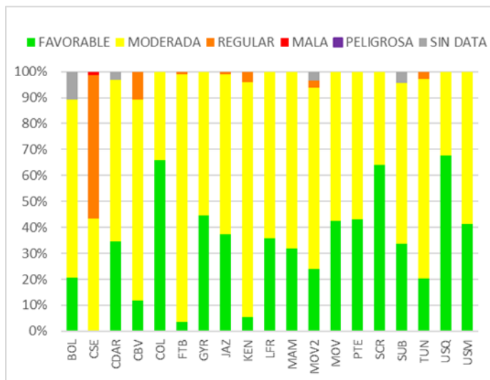
Figura 23. IBOCA para PM 2.5 por estación – octubre 2023
