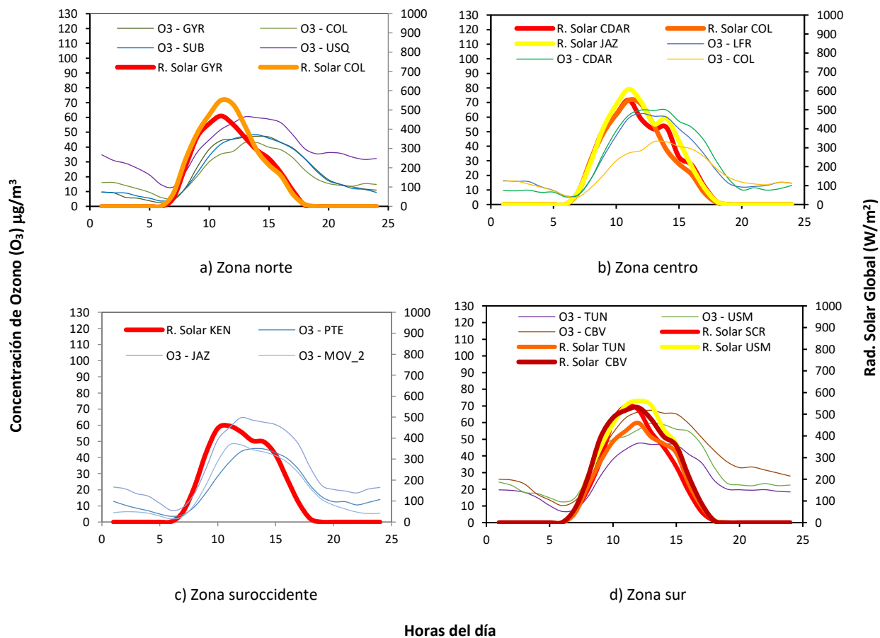
Figura 12. Comportamiento horario de las concentraciones de O_3 ( \mu g/m^3 ) y su relación con la Radiación Solar entrante ( W/m^2 ) octubre 2023. a) zona norte, b) zona centro, c) zona suroccidente y d) zona sur
