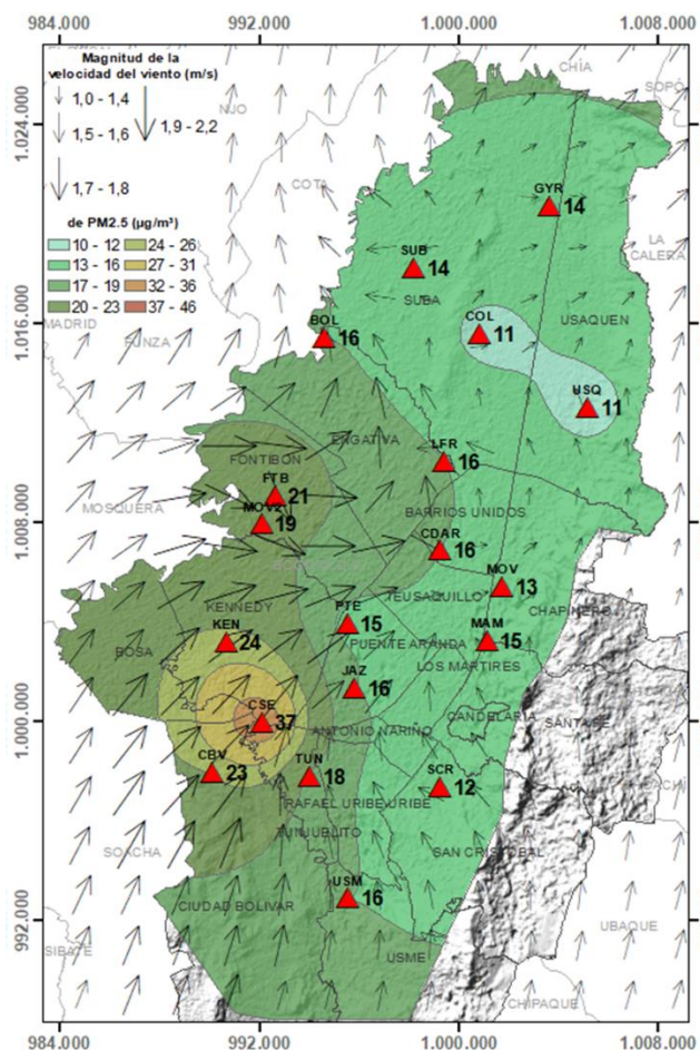
Figura 4. Distribución espacial concentraciones mensuales PM 2.5 – octubre 2023
