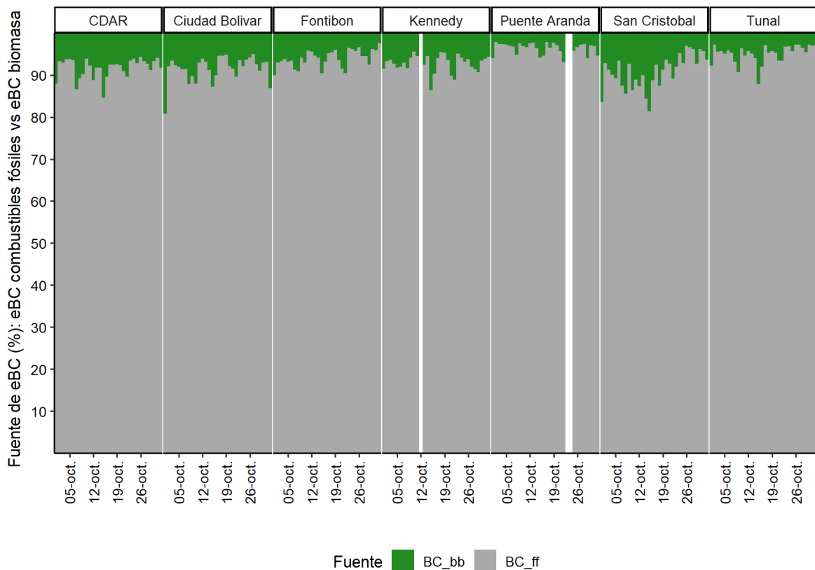
Figura 20. Serie temporal porcentaje de quema Black Carbon de combustibles fósiles BC(ff) vs. Black Carbon de quema de biomasa BC(bb) - octubre de 2023
