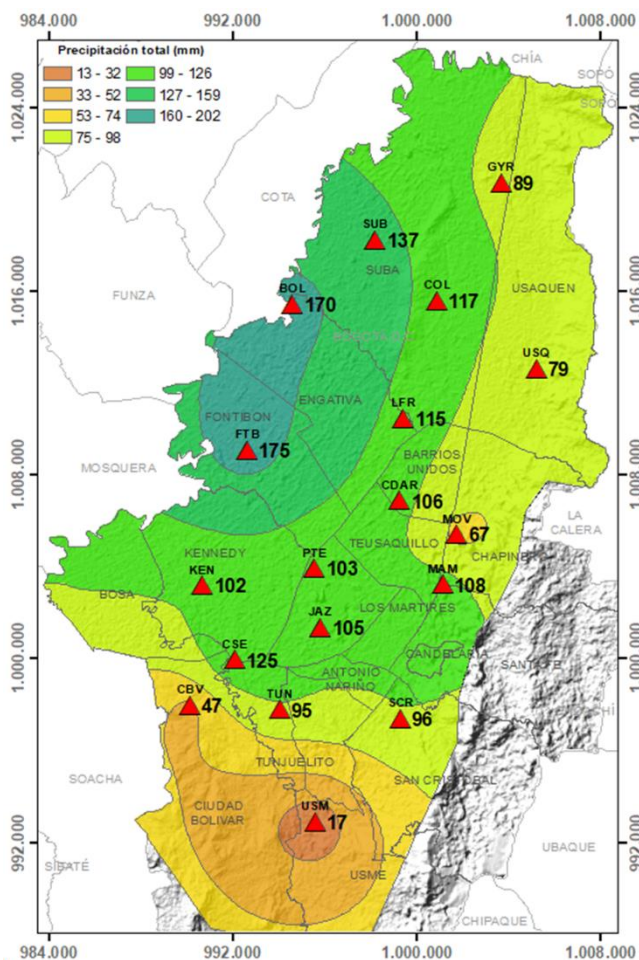
Figura 26. Mapa de la precipitación mensual total (mm) – octubre 2023
