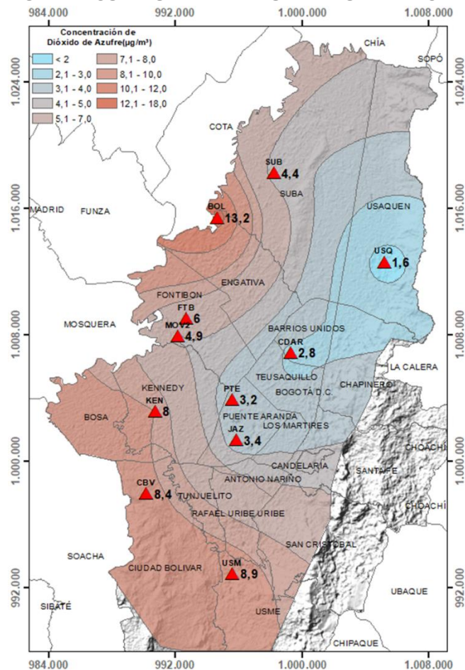
Figura 13. Distribución espacial concentraciones mensuales SO 2 – octubre 2023
