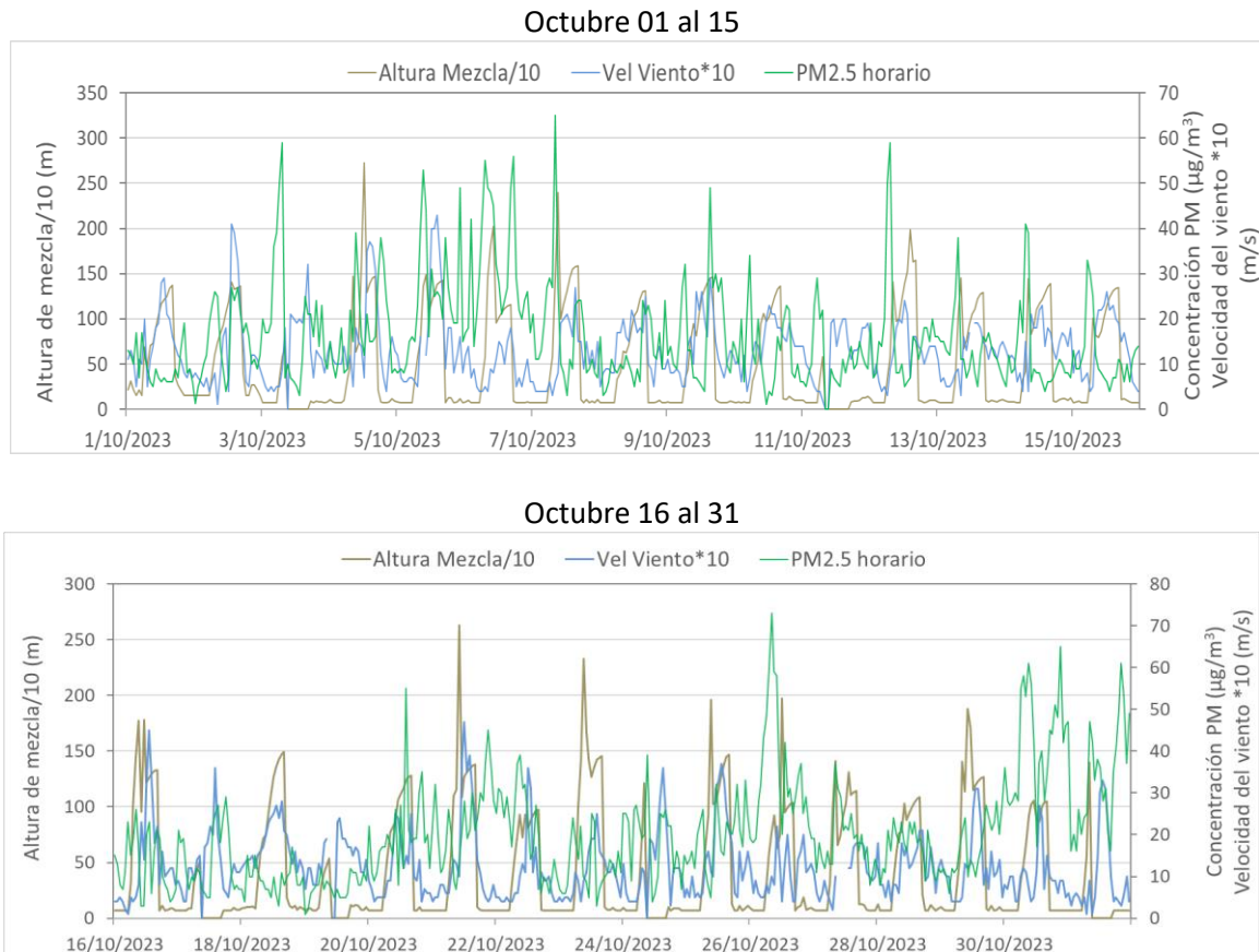
Figura 7. Comparación altura de mezcla, concentraciones PM_{2.5} y velocidad del viento estación Tunal - octubre 2023
