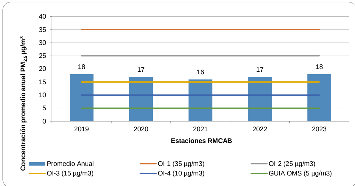
Figura 12-17 Seguimiento a objetivos intermedios de la OMS para exposición anual, para material particulado PM_{2.5} Bogotá 2019 - 2023.
