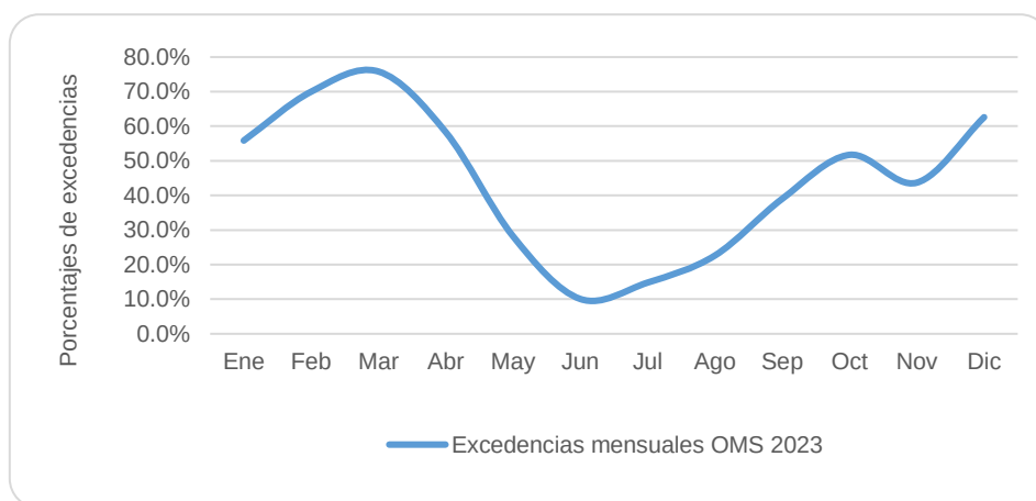
Figura 12-16 Porcentaje de excedencias mensuales, para concentraciones de 24 horas de PM 2,5 , en Bogotá, 2023.
