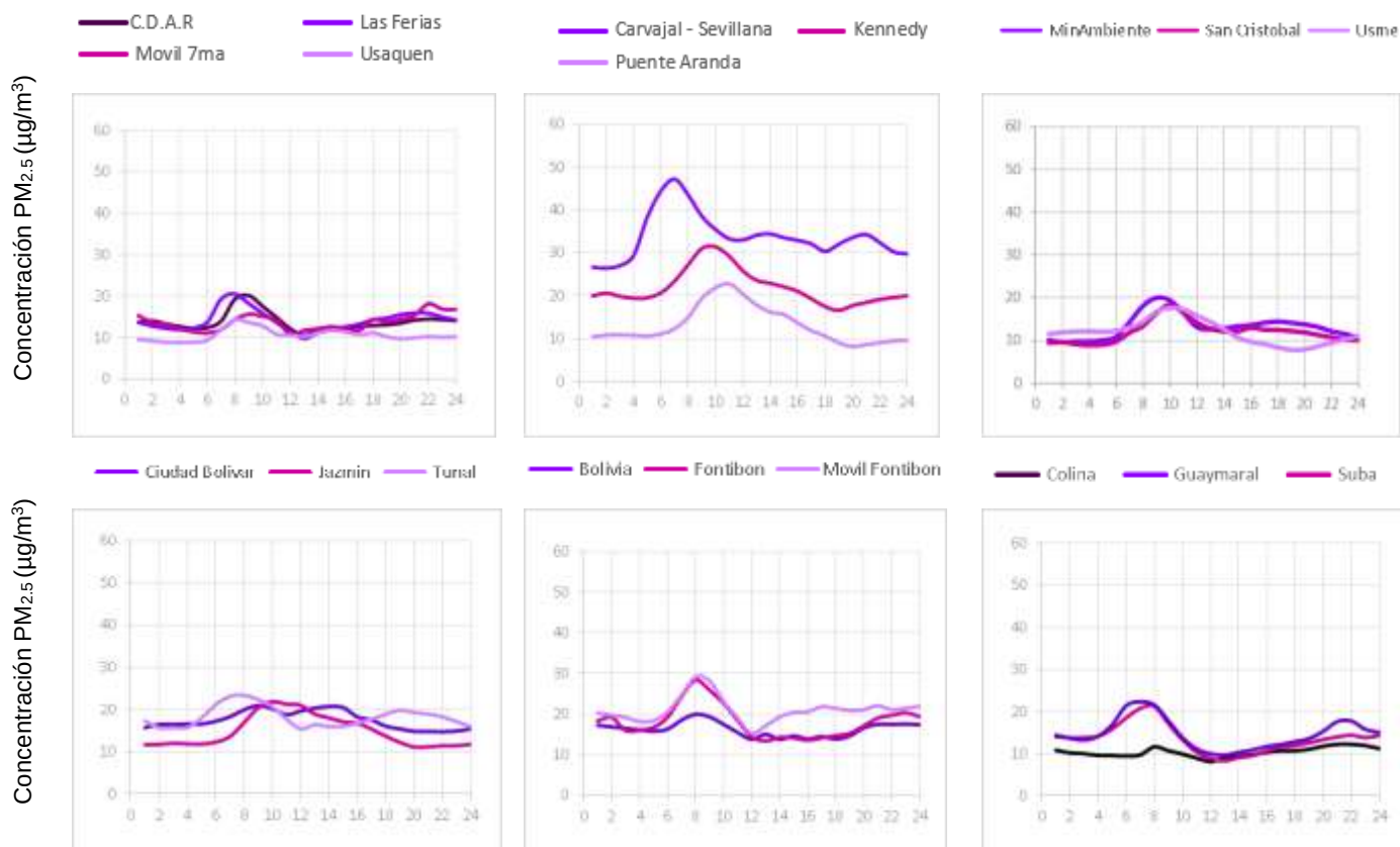
Figura 7-11 Comportamiento horario de las concentraciones de PM_{2.5} – Año 2023
