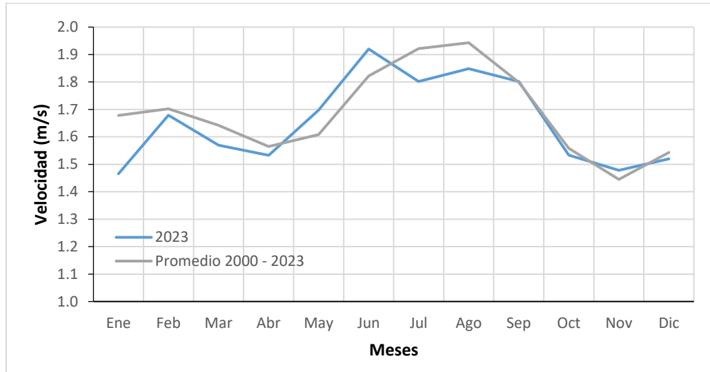
Figura 10 10-13Comportamiento mensual de la velocidad del viento (promedio 2000 – 2023) Vs 2023.
