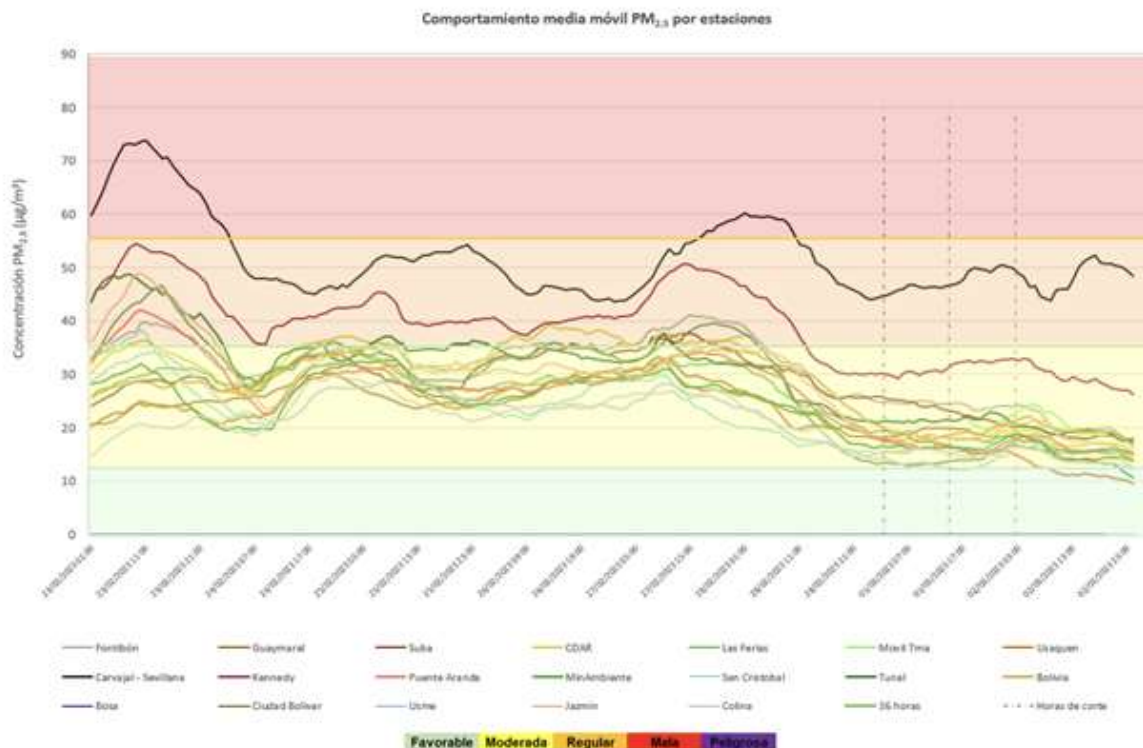
Figura 11-2. Comportamiento concentraciones media móvil 24H PM_{2.5} – alerta fase 1 a nivel ciudad 24 de febrero al 2 de marzo 2023
