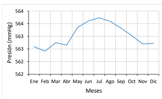
a) Promedio mensual ciudad 2022
