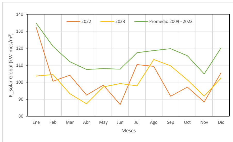
Figura 10 10-21. Comportamiento mensual de la radiación solar en 2022 y 2023 vs. Promedio 2009 - 2023
