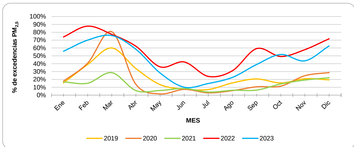
Figura 12-18 Proporción de excedencias de contaminación del aire por material particulado PM_{2.5} respecto a la Guía de Calidad del Aire de la OMS en Bogotá año 2019-2023.
