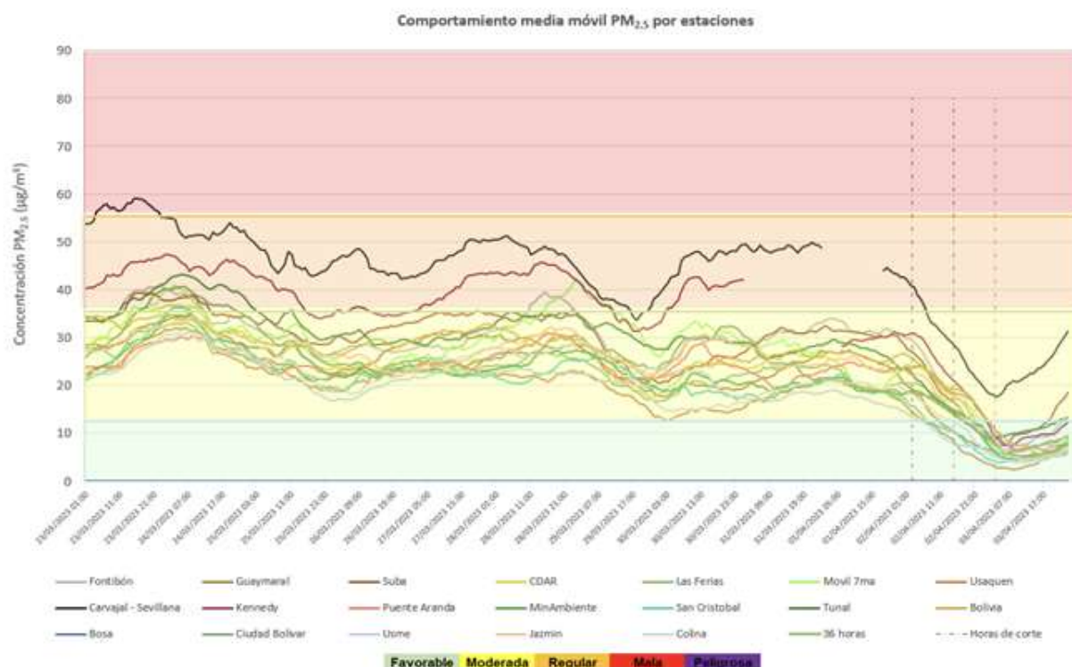
Figura 11-3. Comportamiento concentraciones media móvil 24H PM 2.5 – Alerta Fase 1 Zona Suroccidente 24 de marzo al 3 de abril 2023
