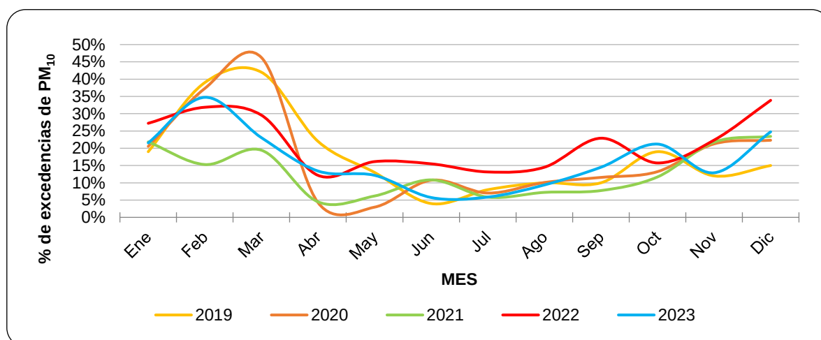
Figura 12-13 Proporción de excedencias de contaminación del aire por material particulado PM 10 respecto a la Guía de Calidad del Aire de la OMS en Bogotá año 2019-2023.
