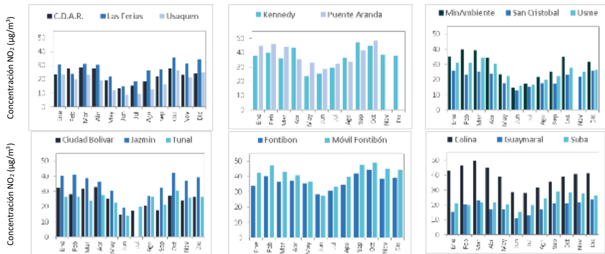
Figura 7-21 Concentraciones mensuales de \text{NO}_2 por estación – Año 2023
