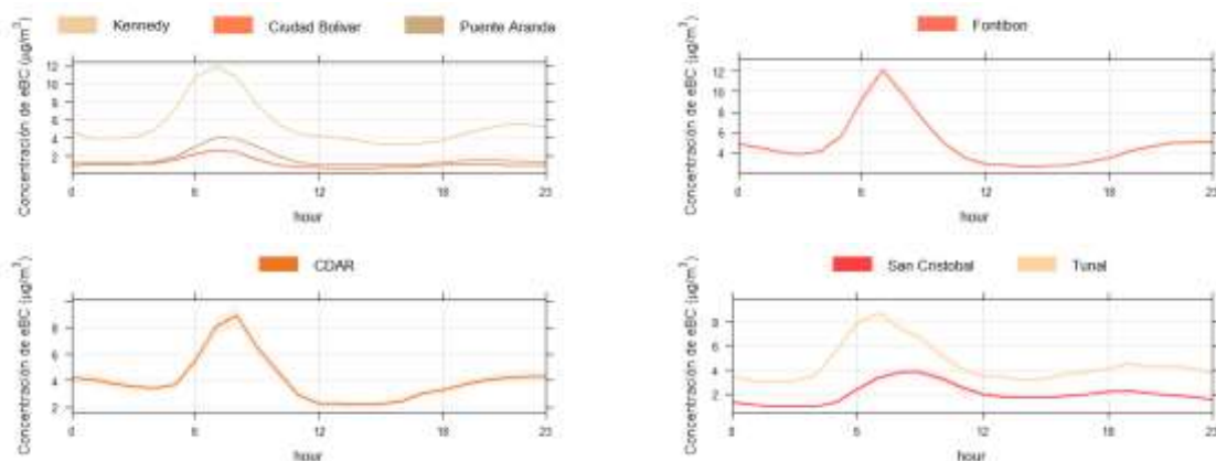
Figura 8-5 Comportamiento horario de las concentraciones de eBC – Año 2023
