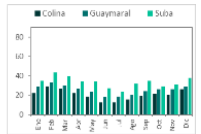
Figura 7-3 Concentraciones mensuales de PM 10 por estación – Año 2023
