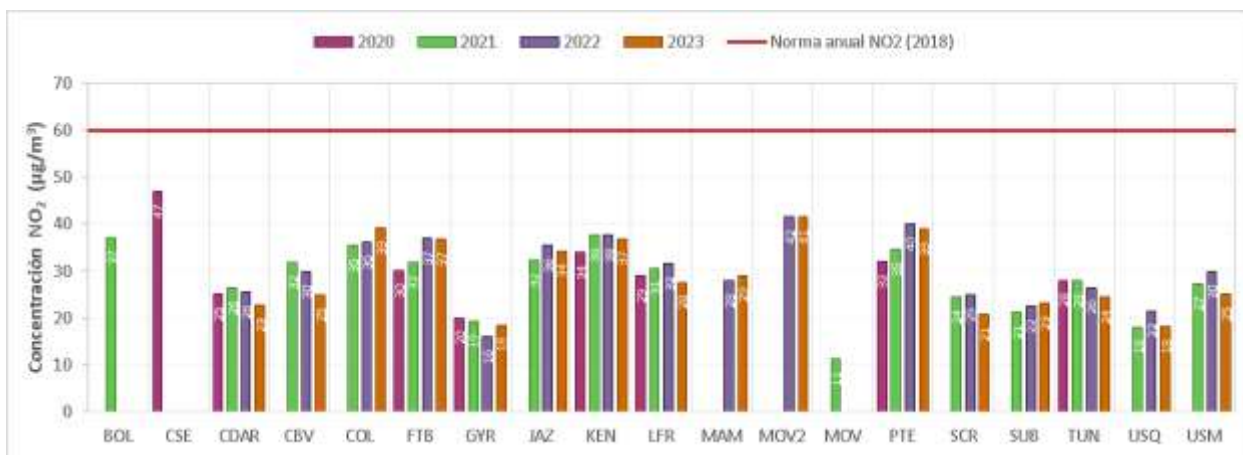
Figura 7-24 Concentraciones promedio anual de NO 2 - Años 2020 a 2023
