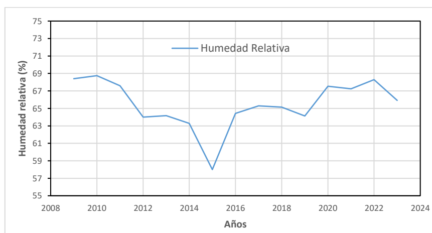
a) Promedio multianual RMCAB 2009 - 2023
