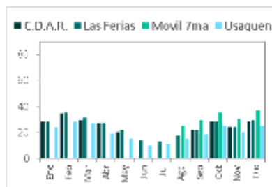
Concentración PM 10 (µg/m 3 )
