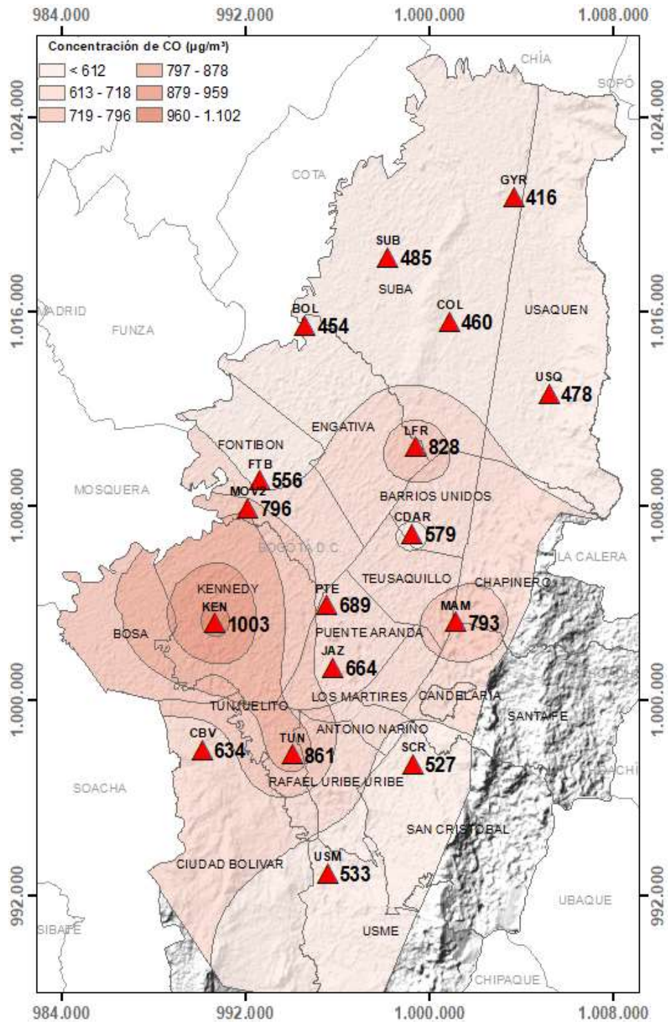
Figura 7-32 Distribución espacial de los promedios anuales de CO del año 2023 con base en el método de interpolación Kriging
