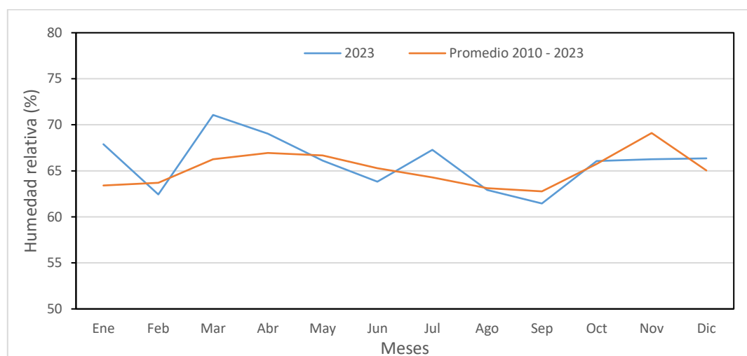
Figura 10 10-29. Comportamiento de la humedad relativa mensual en 2023 Vs promedio mensual multianual 2010-2023
