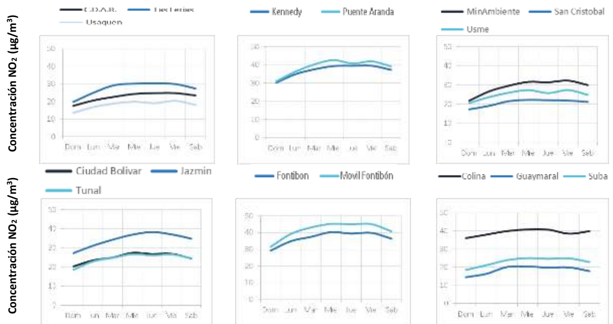
Figura 7-22 Comportamiento diario de las concentraciones de \text{NO}_2 – Año 2023
