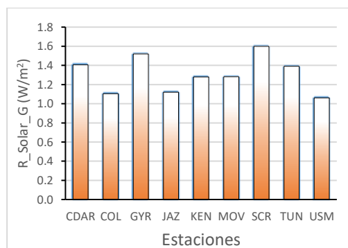
b) Acumulado por estación
