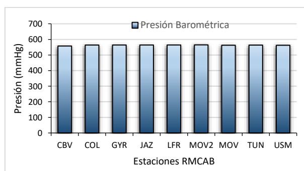
b) Promedio anual por estación 2022
