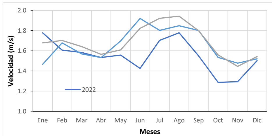
Figura 10 10-15. Comportamiento de la velocidad media mensual en 2022 y 2023 Vs. promedio mensual multianual 2000 - 2023
