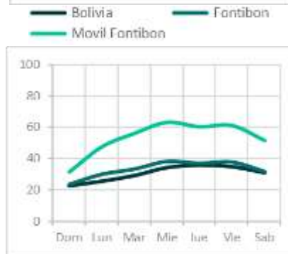
Figura 7-4 Comportamiento diario de las concentraciones de PM 10 – Año 2023
