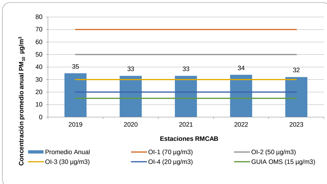
Figura 12-12 Seguimiento a objetivos intermedios de la OMS, para exposición anual, de PM 10 Bogotá 2019-2023.
