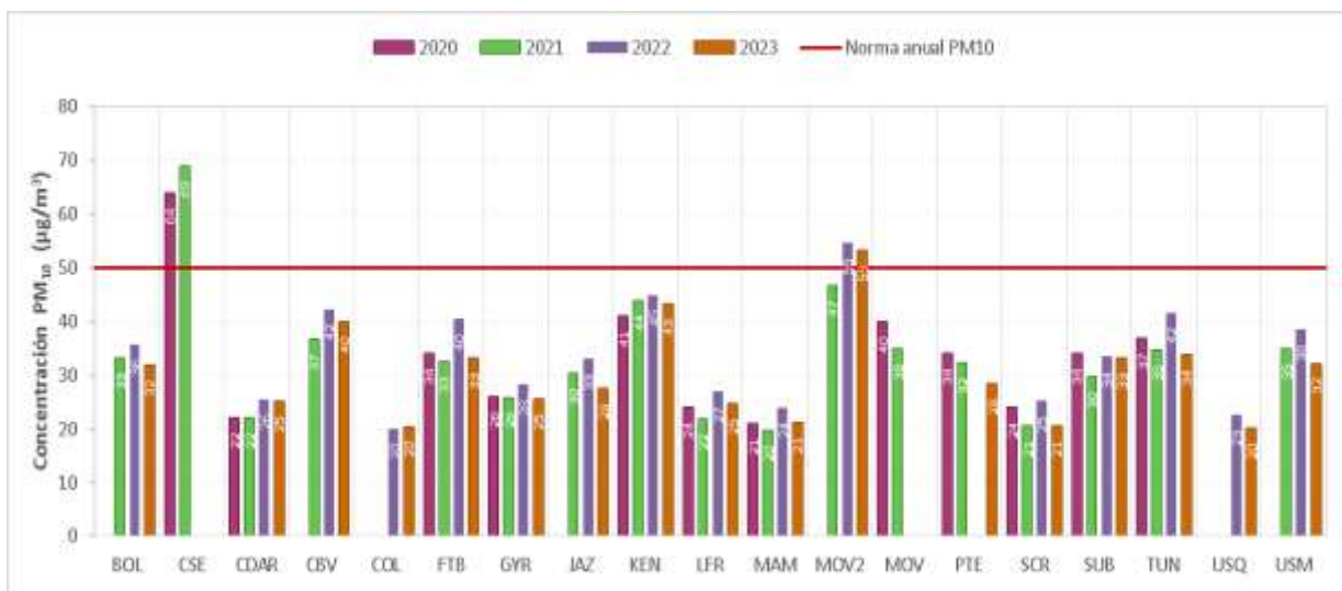
Figura 7-6 Concentraciones anuales de PM10 años 2020 a 2023
