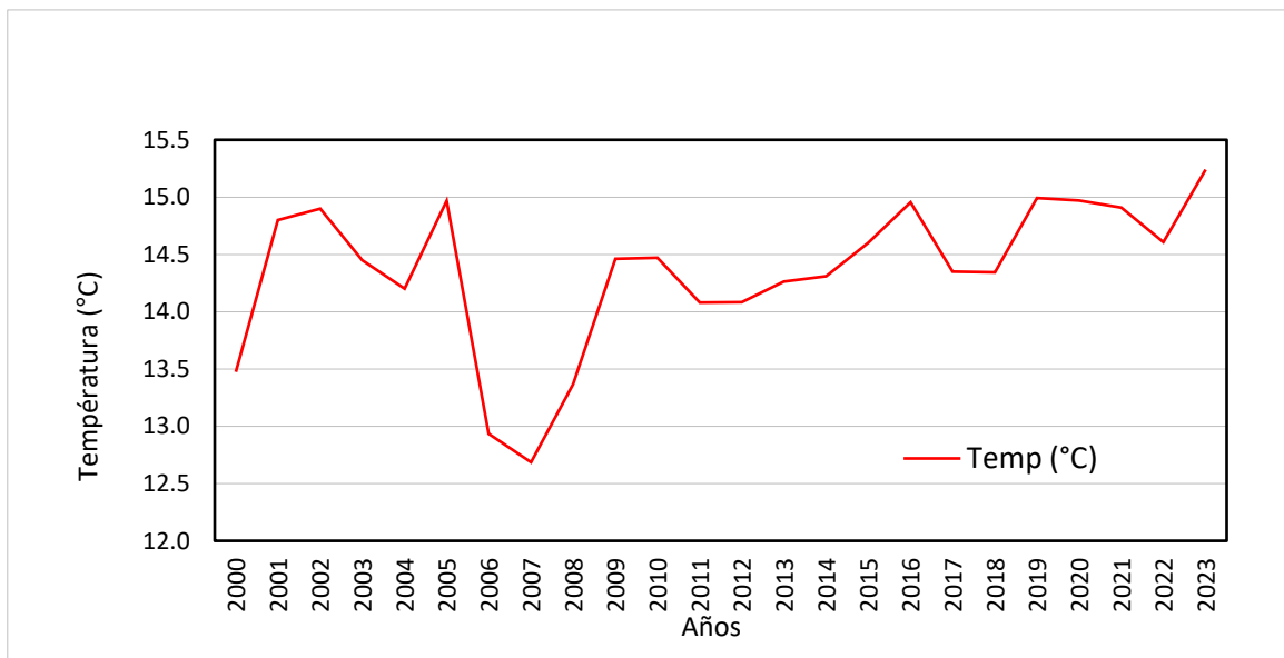
Figura 10-10-12. Comportamiento histórico de la temperatura desde 2000 a 2023
