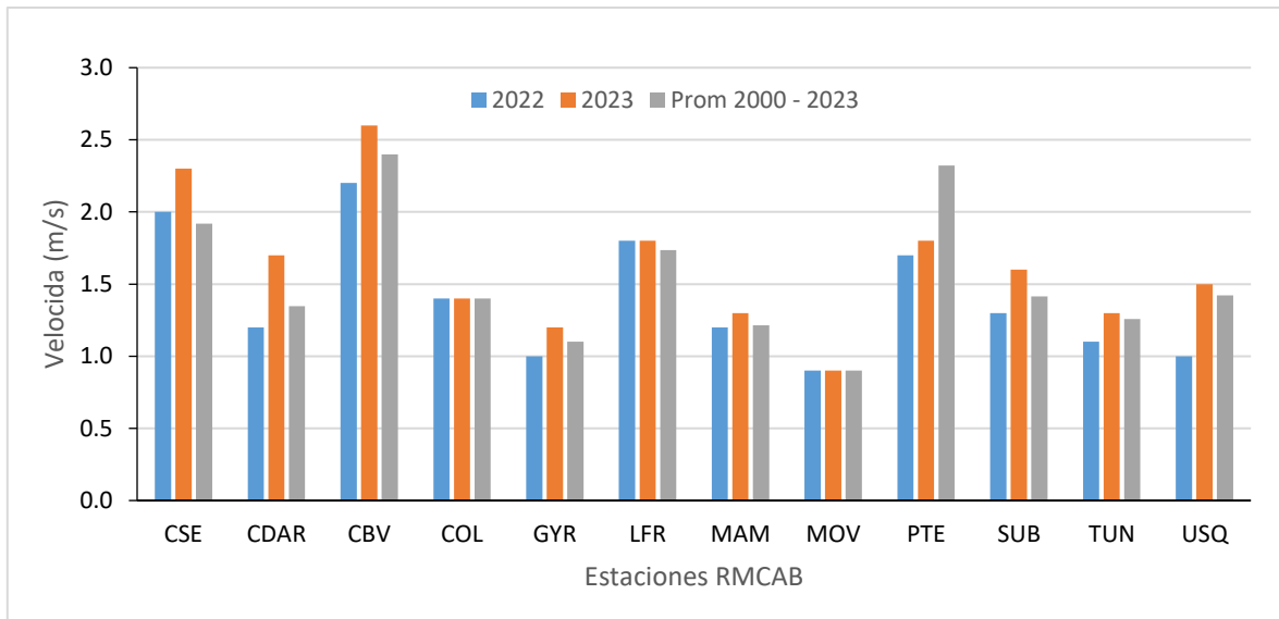
Figura10 10-14 Comportamiento de la velocidad del viento promedio anual 2022, 2023 Vs (2000 – 2023).
