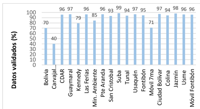
Figura 6-4 Porcentaje de datos válidos por estación - Año 2023
