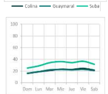
Figura 7-4 Comportamiento diario de las concentraciones de PM 10 – Año 2023
