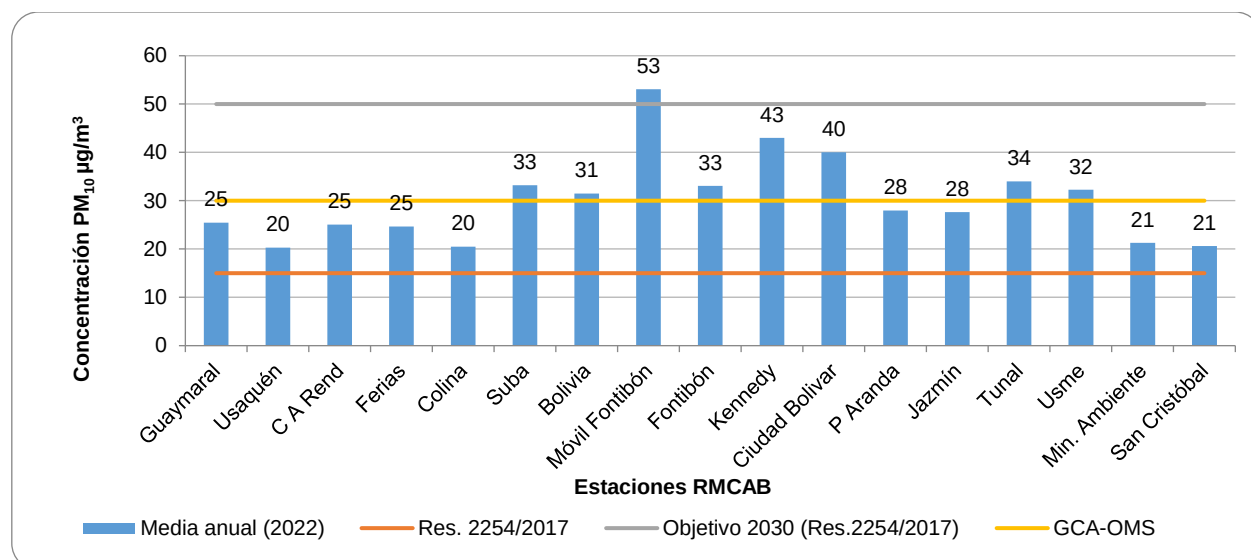
Figura 12-9 Concentración promedio y excedencia a la normativa Guía-OMS y Resolución 2254 de 2017 de PM 10 , para estaciones de la RMCAB, 2023.
