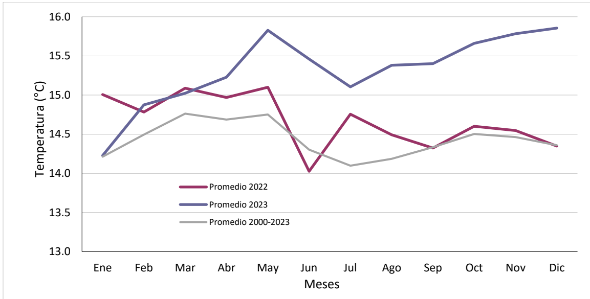
Figura 10-10-8. Comportamiento de la temperatura mensual multianual periodo 2000-2023 Vs 2022 y 2023
