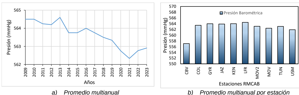
Figura 10 10-28. Comportamiento de la presión atmosférica promedio multianual 2009 - 2023
