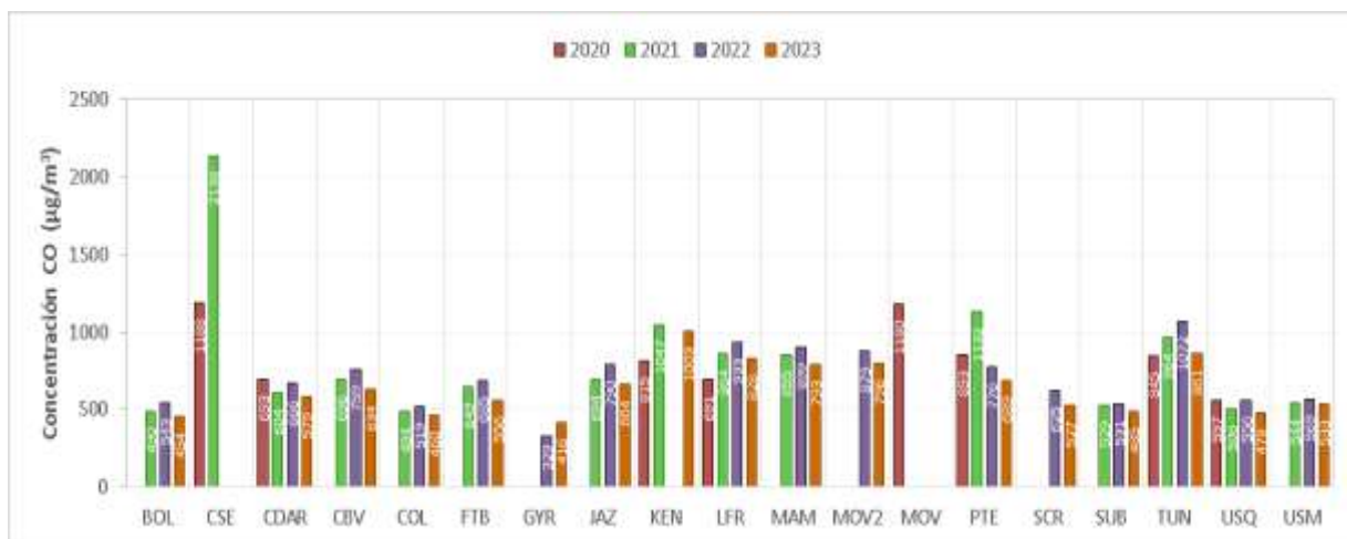
Figura 7-36 Concentraciones anuales de CO años 2020 a 2023
