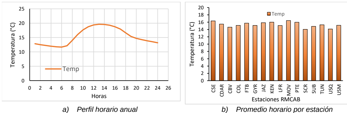
Figura 10-10-7. Comportamiento de la temperatura horaria anual-2023: a) perfil horario; b) promedio por estación
