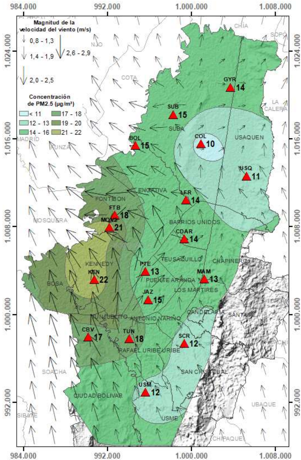
Figura 7-8 Distribución espacial de los promedios anuales de PM 2.5 del año 2023 con base en el método de interpolación Kriging
