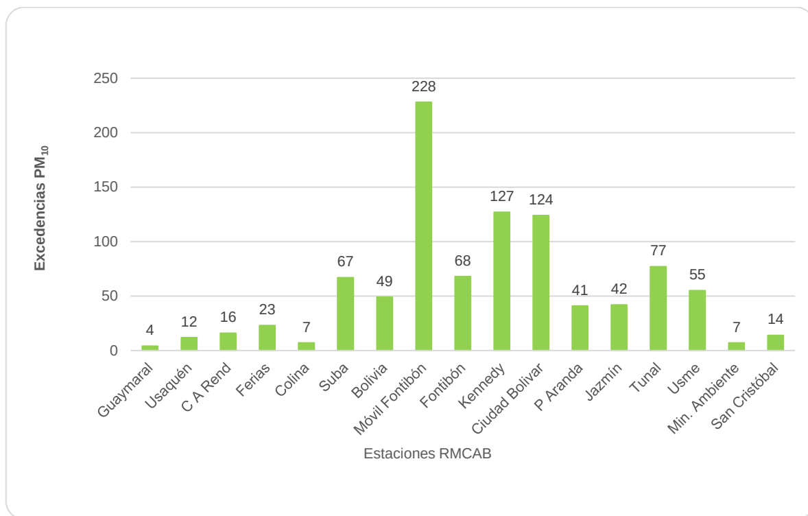
Figura 12-10 Excedencias de concentraciones de PM 10 , respecto a la Guía-OMS en las estaciones de la RMCAB, 2023.
