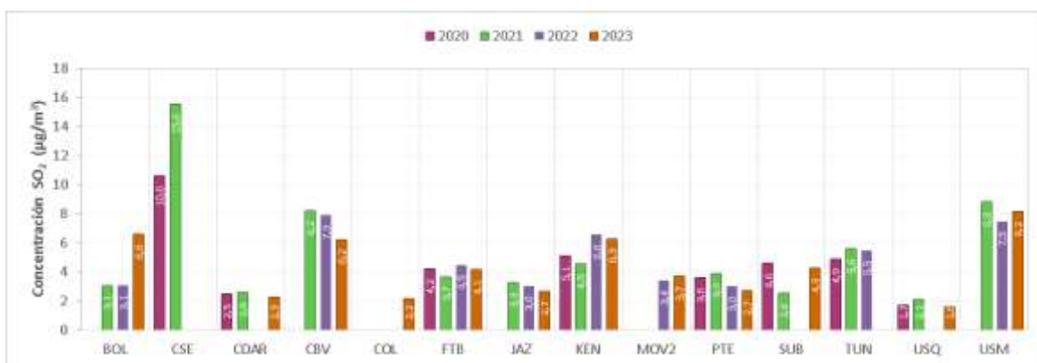
Figura 7-30 Concentraciones anuales de \text{SO}_2 años 2020 a 2023
