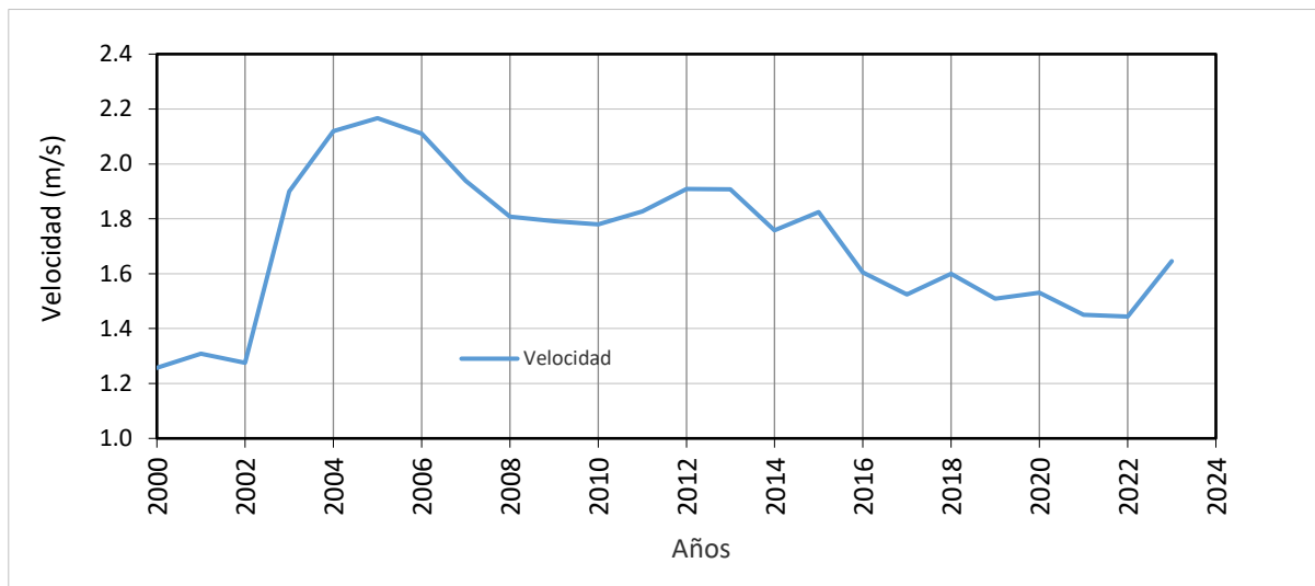
Figura 10 10-20 Comportamiento medio multianual de la velocidad del viento en Bogotá entre 2000 a 2023
