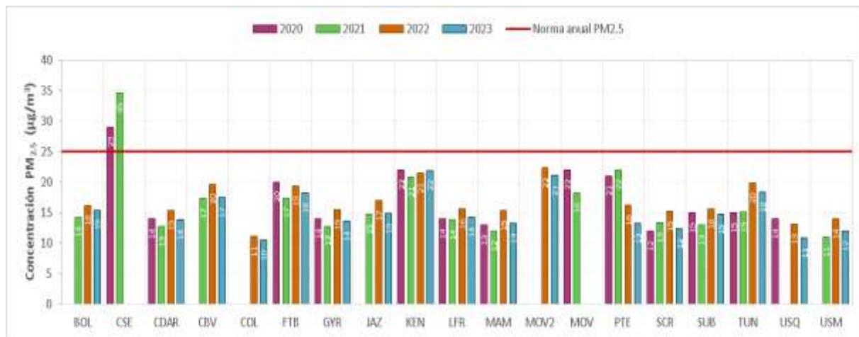
Figura 7-12 Concentraciones anuales de PM 2.5 años 2020 a 2023
