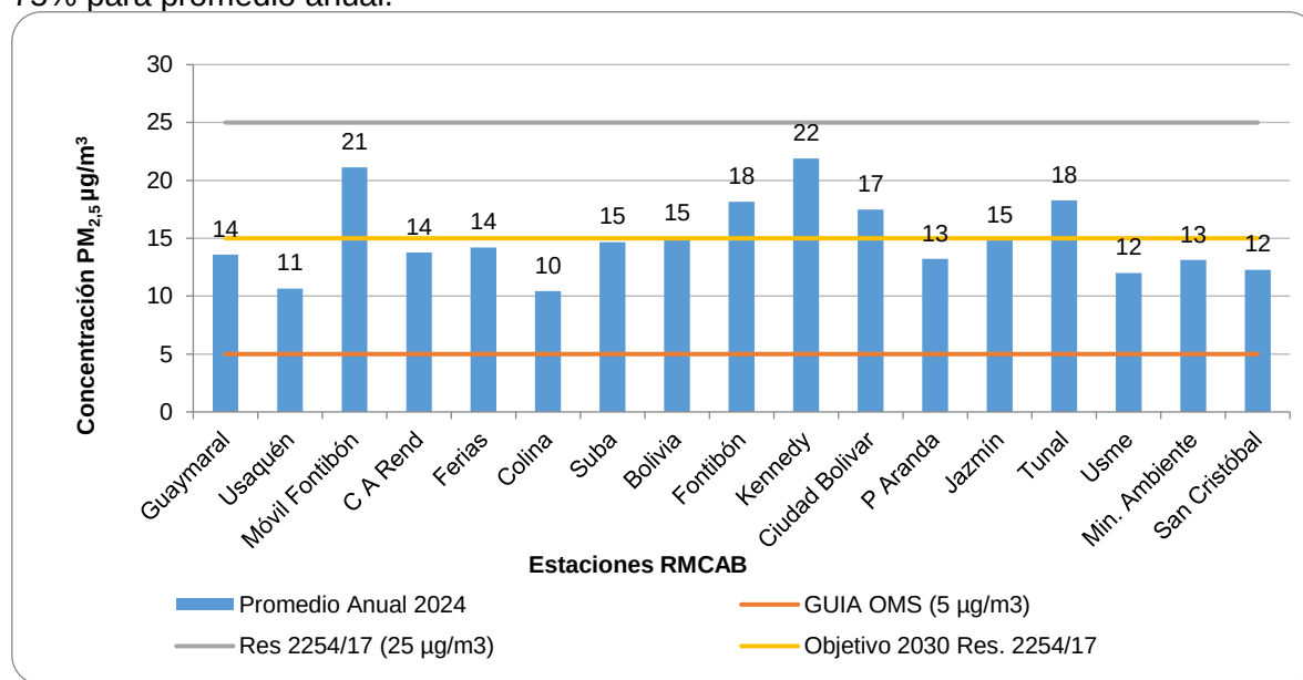
Figura 12-14 Concentración promedio y excedencia a la normativa Guía-OMS y Resolución 2254 de 2017 de PM 2.5 para estaciones de la RMCAB, 2023.
