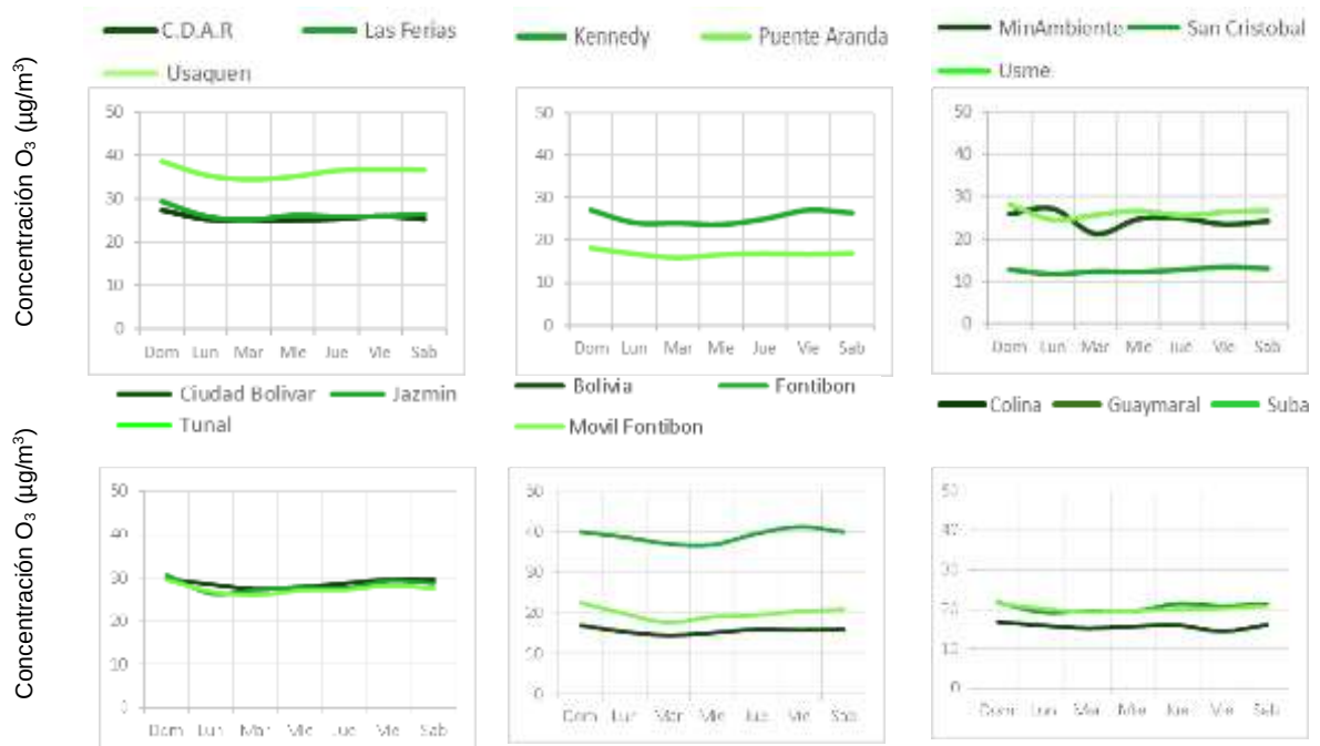
Figura 7-16 Comportamiento diario de las concentraciones de O_3 – Año 2023
