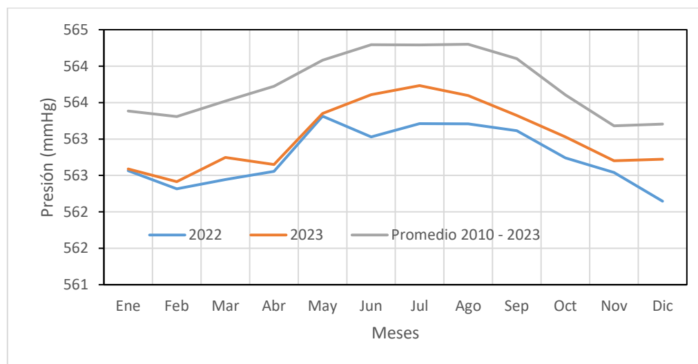
Figura 10 10-25. Comportamiento mensual de la presión en 2022 y 2023 frente al promedio mensual multianual 2010-2023
