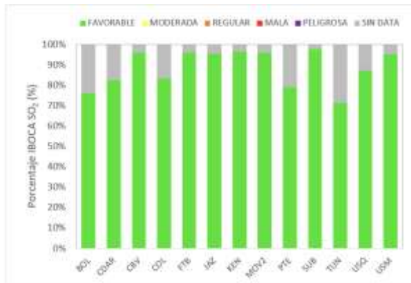
Figura 9-4 IBOCA por estación de monitoreo para O 3 , NO 2 , SO 2 y CO – Año 2023
