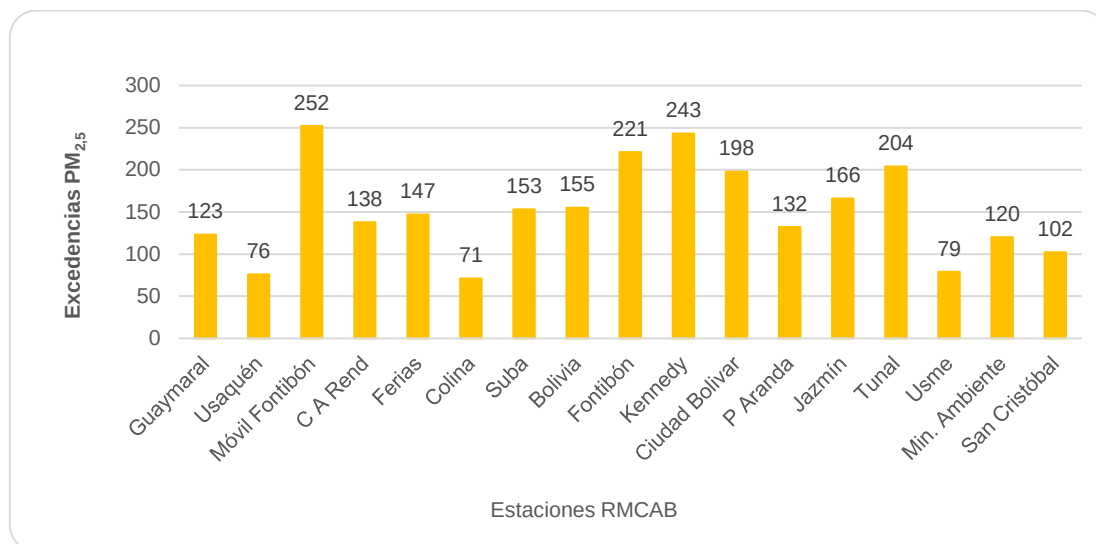
Figura 12-15 Excedencias de PM 2,5 , respecto a la Guía-OMS en las estaciones de la RMCAB, 2023.
