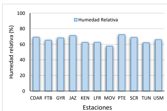
b) Promedio por estación 2023 c)
