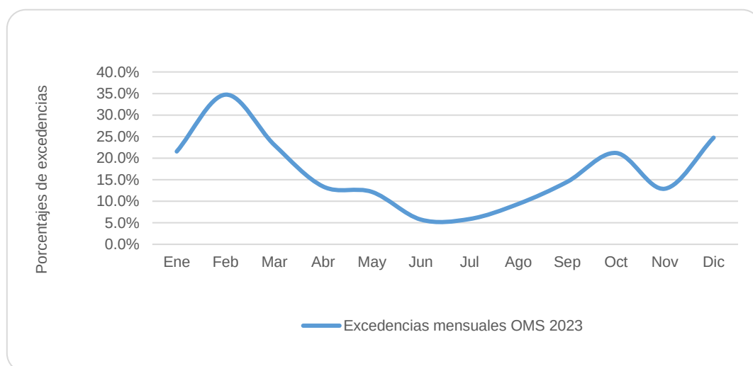
Figura 12-11 Porcentaje de excedencias mensuales, para concentraciones de 24 horas de PM 10 , en Bogotá, 2023.
