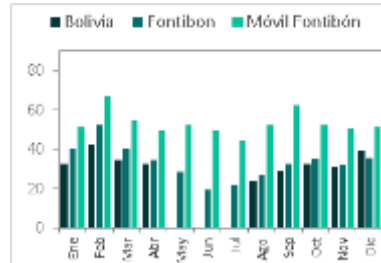
Figura 7-3 Concentraciones mensuales de PM 10 por estación – Año 2023
